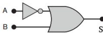
Figura 4.11: Exemplo NOT e OR.
