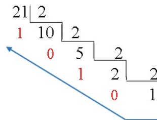
Figura 4.5: Converter 21_{10} para binário.
