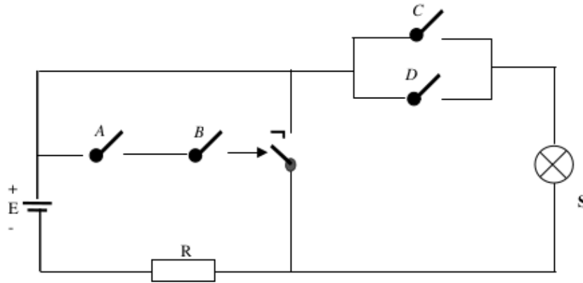
Figura 4.13: Circuito de chaveamento.
