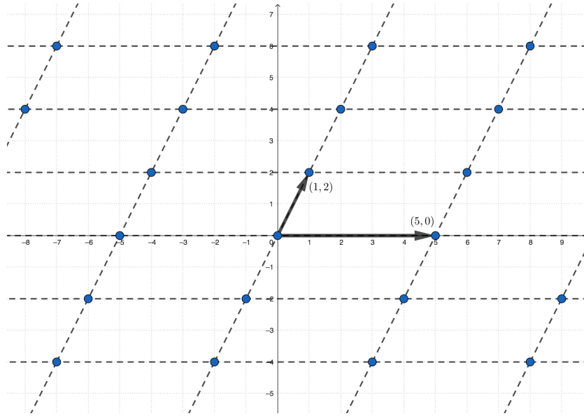
Figura 7 – Reticulado \Lambda_2 .
