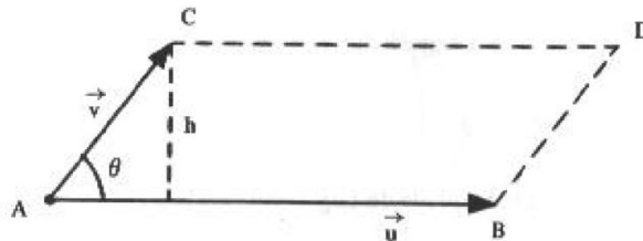
Figura 3 – Interpretação Geométrica do Produto Vetorial.
