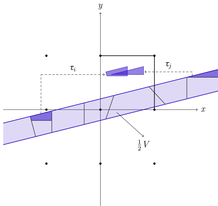
Figura 12 – Intersecção não vazia de (U_i + i) e (U_j + j) .
