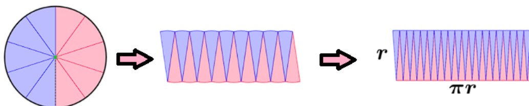
Figura 1.5 – Construção da área do círculo
