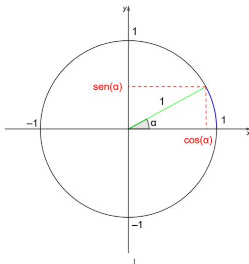
Figura 1.10 – Seno e cosseno
