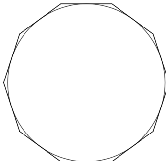
Figura 1.4 – Polígono inscrito na circunferência
