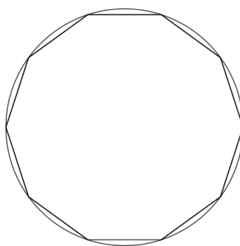
Figura 1.3 – Polígono inscrito na circunferência
