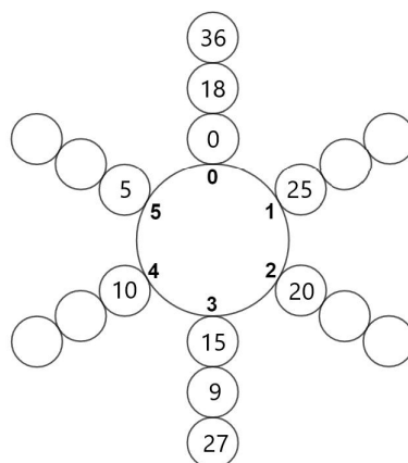
Figura 1.16 – Preenchimento dos valores relativos a cada resíduo módulo 6.
