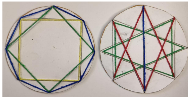
Figura 1.2 – Exemplos de construções com m = 8 e m = 10 .
