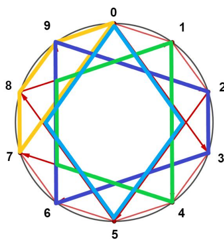
(c) Alguns quadriláteros encontrados.
