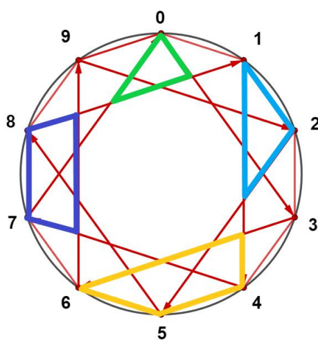
(b) Alguns triângulos e quadriláteros encontrados.
