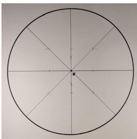
(c) Oito pontos.
