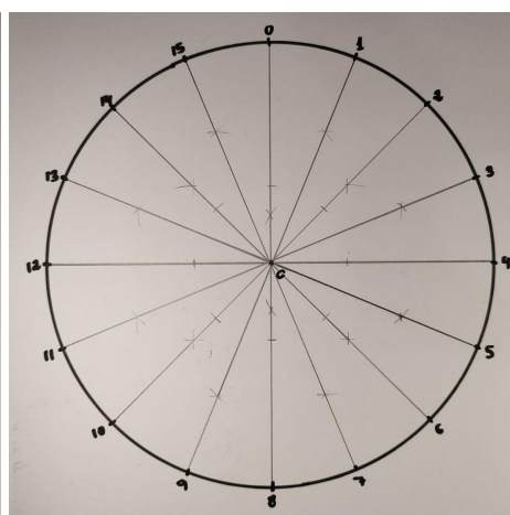
(d) Dezesesseis pontos.
