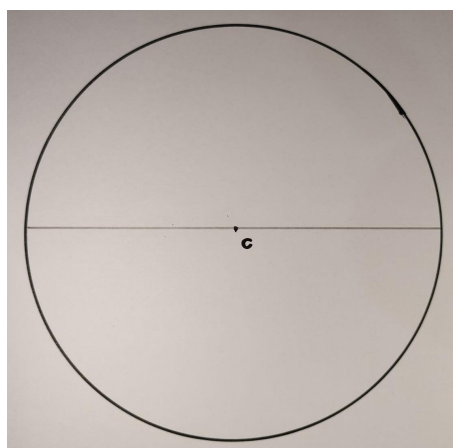
(a) Dois pontos.
