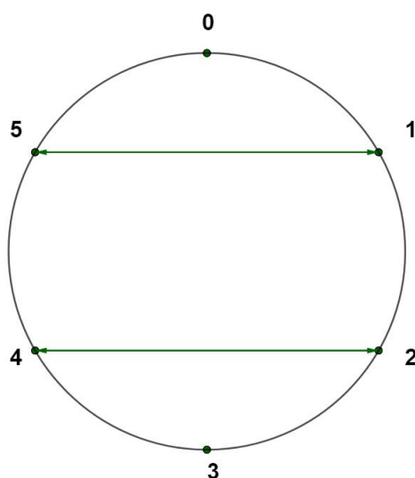
Figura 1.13 – Chryzode de multiplicação por 5, módulo 6.
