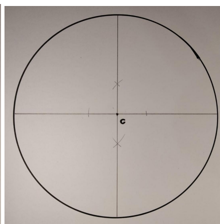
(b) Quatro pontos.
