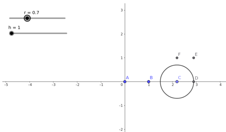
Figura 4.9: Construção no GeoGebra (Padrões moiré ) I
