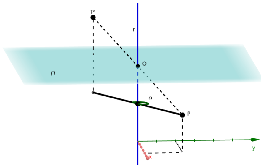
Figura 3.10: Rotação refletida II
