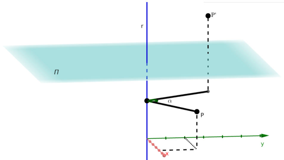
Figura 3.9: Rotação refletida I
