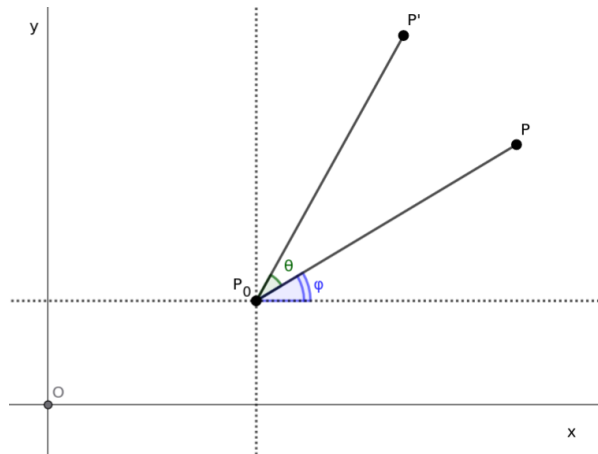
Figura 3.11: Rotação de ângulo \theta em torno de um ponto P_0
