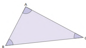
Figura 10 – Triângulo ABC
