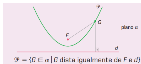
Figura 14 – Parábola \mathcal{P}
