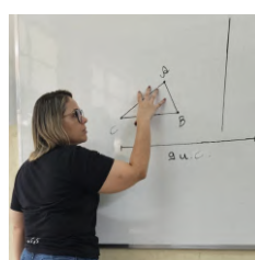
(a) Polígono
