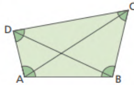
Figura 11 – Quadrilátero ABCD
