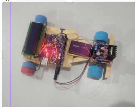
Figura 8 – Carrinho híbrido montado.
