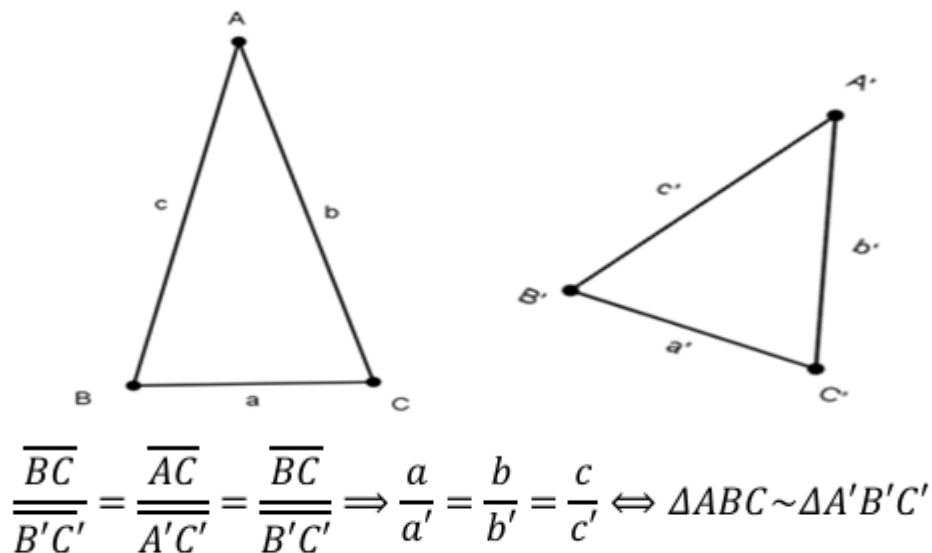
Figura 11 - Triângulos Semelhantes caso LLL
