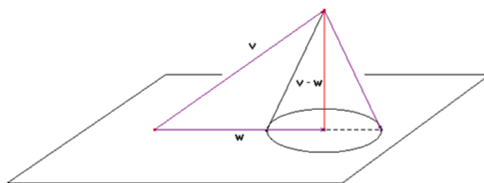
Figura 3.5: a distância é mínima se tomarmos a projeção sobre a perpendicular
