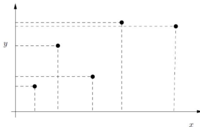
Figura 3.1: Exemplo ilustrativo de um diagrama de dispersão
