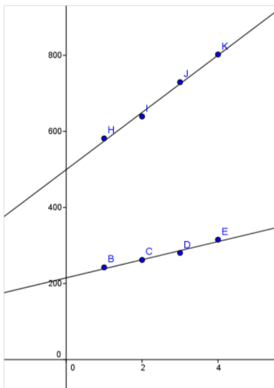
Figura 4.10: Retas y = 23,8x + 215,5 e y = 75,3x + 499,5
