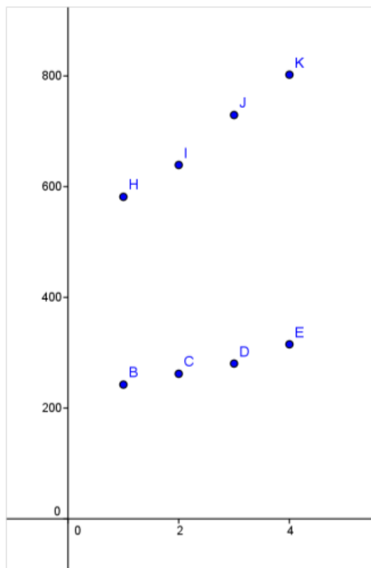
Figura 4.7: gráfico apresenta o valor destas duas grandezas em função do ano em que foram estabelecidas
