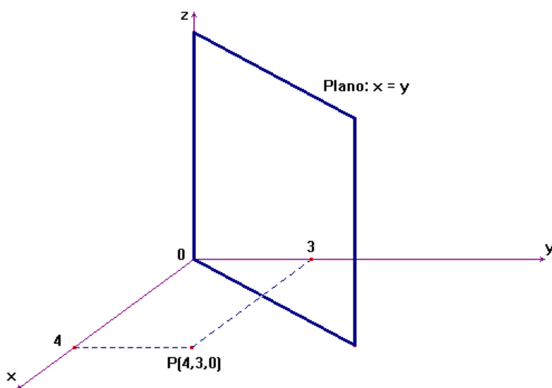
Figura 4.1: O terno (4, 3, 0) do sistema original não pertence ao plano x = y
