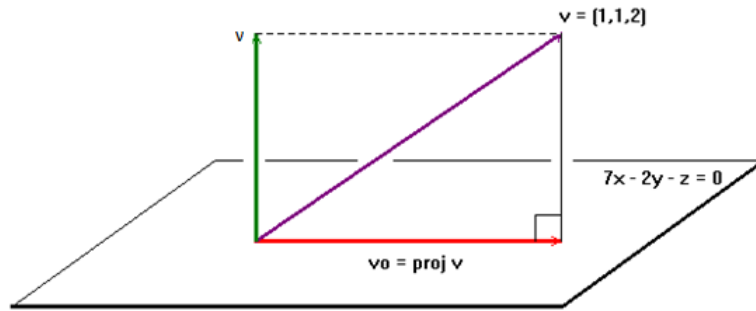
Figura 3.7: projeção ortogonal do vetor v(1, 1, 2) sobre o plano \pi : 7x - 2y - z = 0
