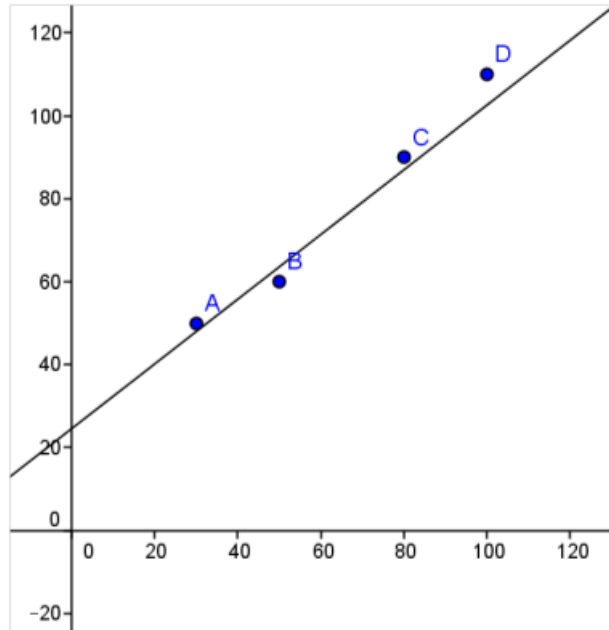
Figura 3.11: pontos resultantes da experiência no plano cartesiano
