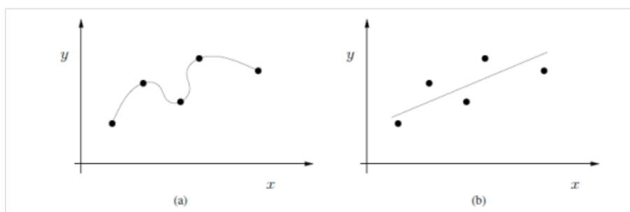
Figura 3.9: Exemplos ilustrativos de uma curva polinomial interpoladora (a) e uma curva que se ajusta aos pontos de um diagrama de dispersão (b)
