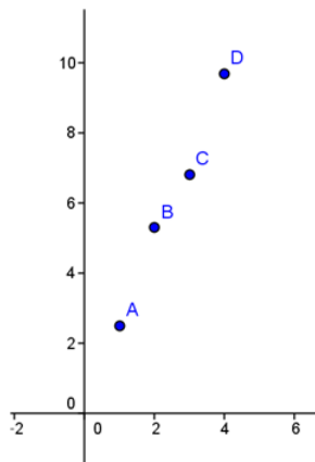
Figura 2.4: Disposição dos pares ordenados (x, y) no plano cartesiano
