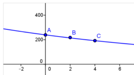
Figura 3.18: Gráfico da função que descreve o número de onças pintadas na região
