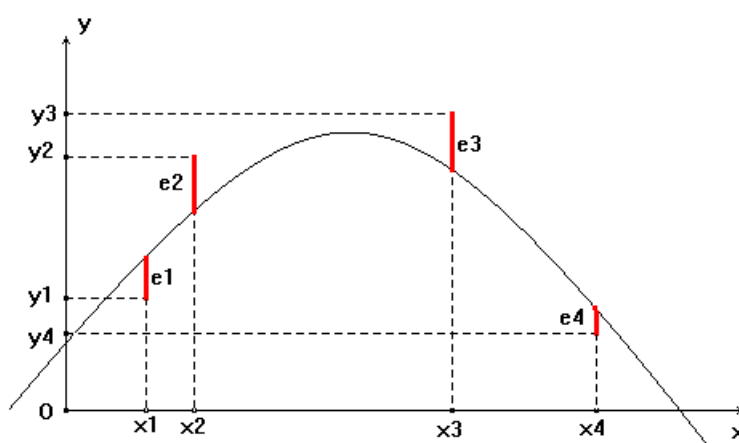
Figura 3.15: diferença ou erro na direção vertical
