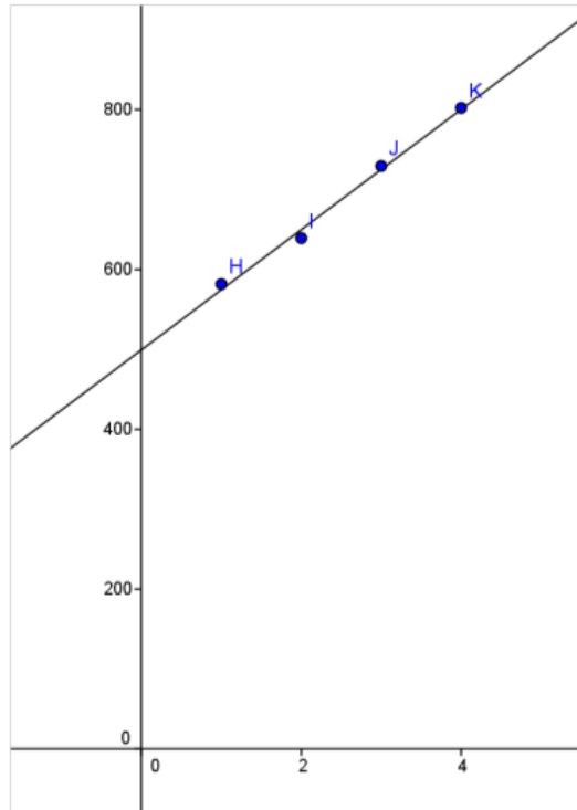
Figura 4.9: Reta y = 75,3x + 499,5
