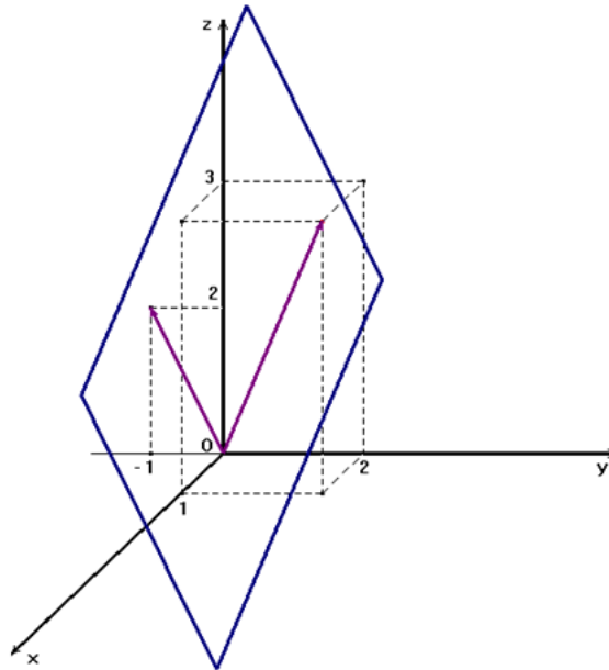
Figura 3.4: Plano W : 7x - 2y - z = 0
