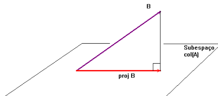
Figura 3.8: A\bar{X} = proj_{col(A)} B
