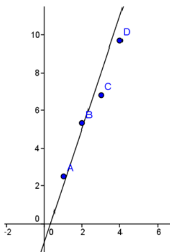
Figura 2.5: Proximidade dos pontos à função afim: f(x) = 3x - 1
