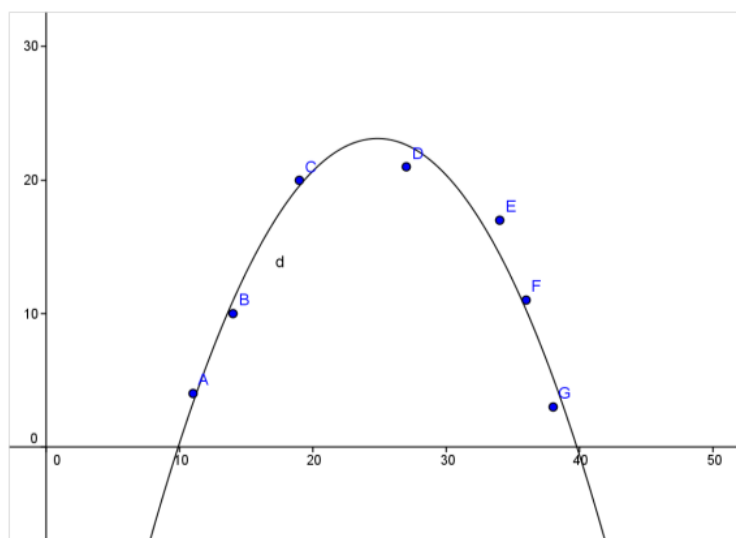
Figura 3.13: Gráfico da função do tipo “ P = aQ^2 + bQ + c ”
