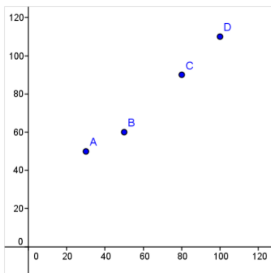
Figura 4.5: gráfico de dispersão desse experimento
