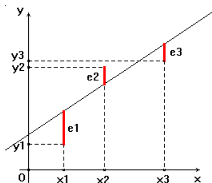
Figura 3.14: Gráfico de e_i
