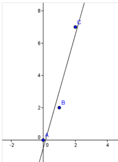
Figura 4.4: Reta y = \frac{7}{2}x - \frac{1}{2}
