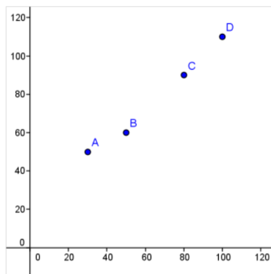
Figura 3.10: gráfico de dispersão desse experimento
