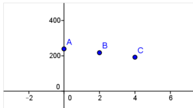
Figura 3.17: Gráfico dos pontos A,B e C
