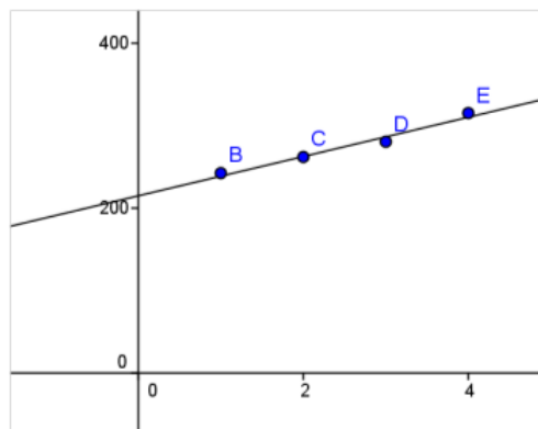
Figura 4.8: Reta y = 23,8x + 215,5
