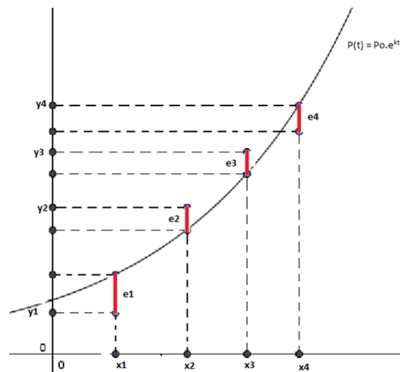
Figura 3.16: diferença ou erro na direção vertical
