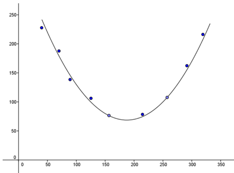
Figura 3.3: Curva que melhor se aproxima do modelo em questão
