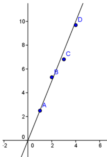
Figura 2.6: Gráfico da função linear definida por: f(x) = 2,5x
