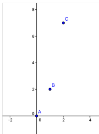
Figura 4.3: Pontos A(0,0) , B(1,2) e C(2,7)
