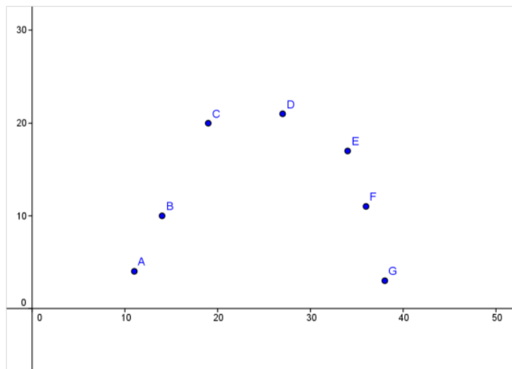
Figura 3.12: pontos resultantes da experiência da medição de P e Q
