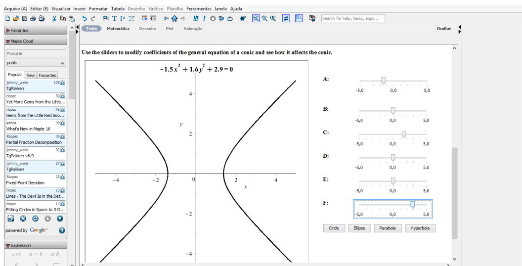
Figura 27 – Variação da distância focal da hipérbole cujo eixo transverso é o OX
