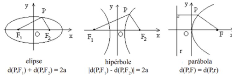
Figura 2 – Gráficos da elipse, hipérbole e parábola e disposição dos eixos coordenados em relações aos quais suas equações são reduzidas.
