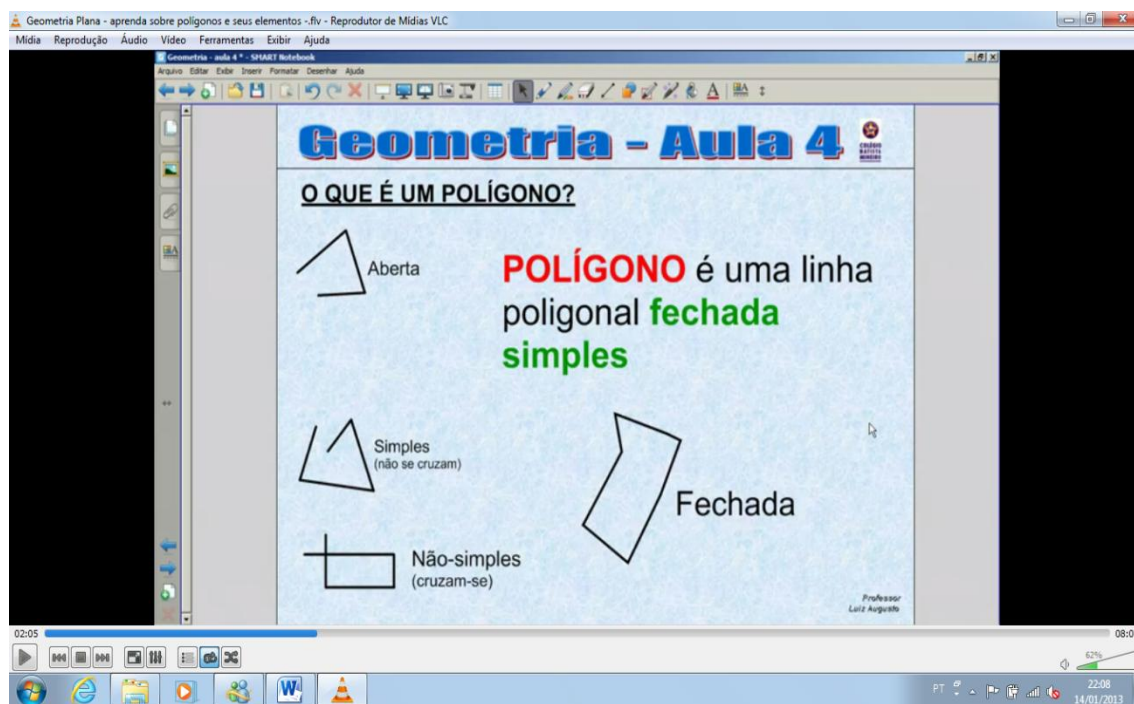
Figura 14: Aprendendo Polígonos
