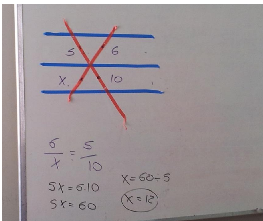
Figura 26: Exemplos para estudo do Teorema de Thales
