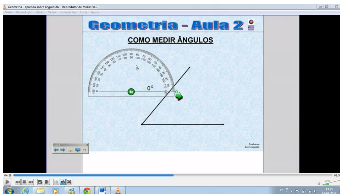
Figura 10: Estudo sobre ângulos
