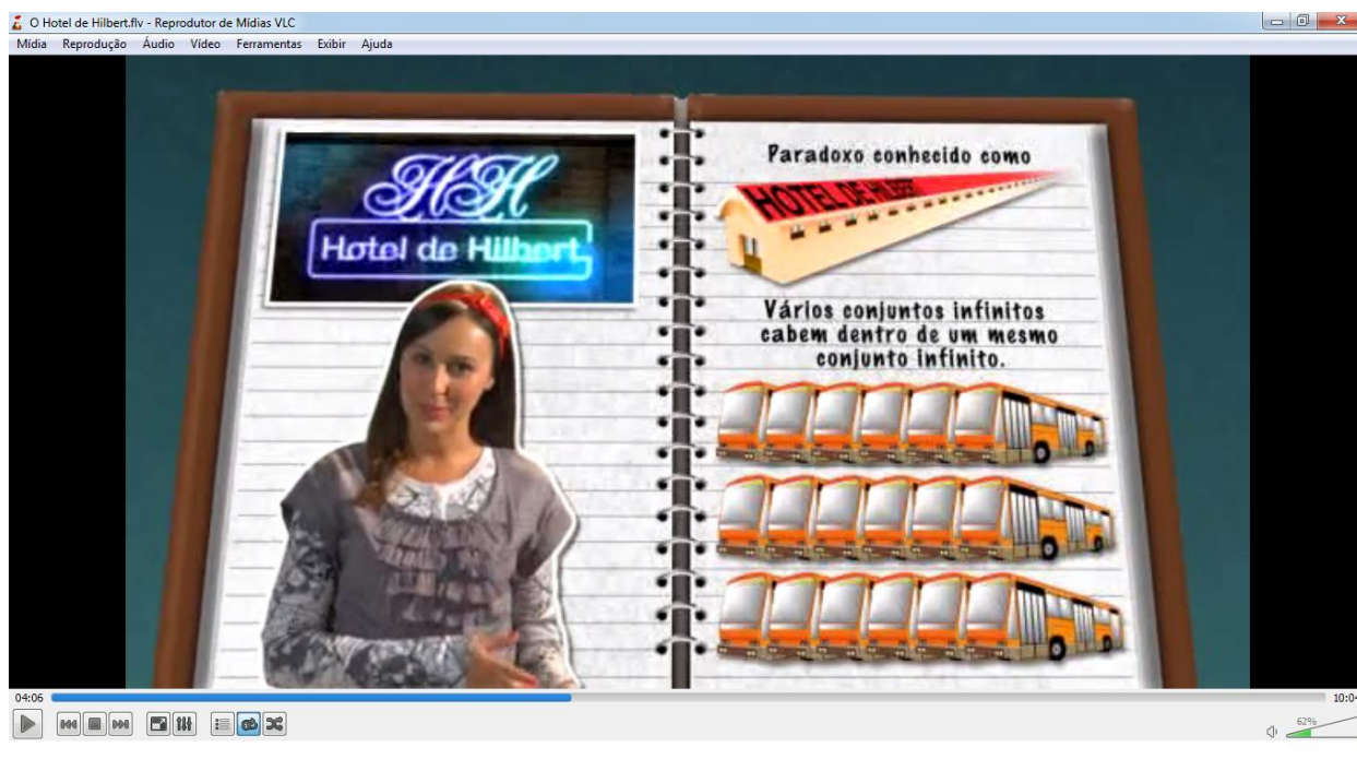
Figura 21: Aprendendo o Conceito do Infinito
