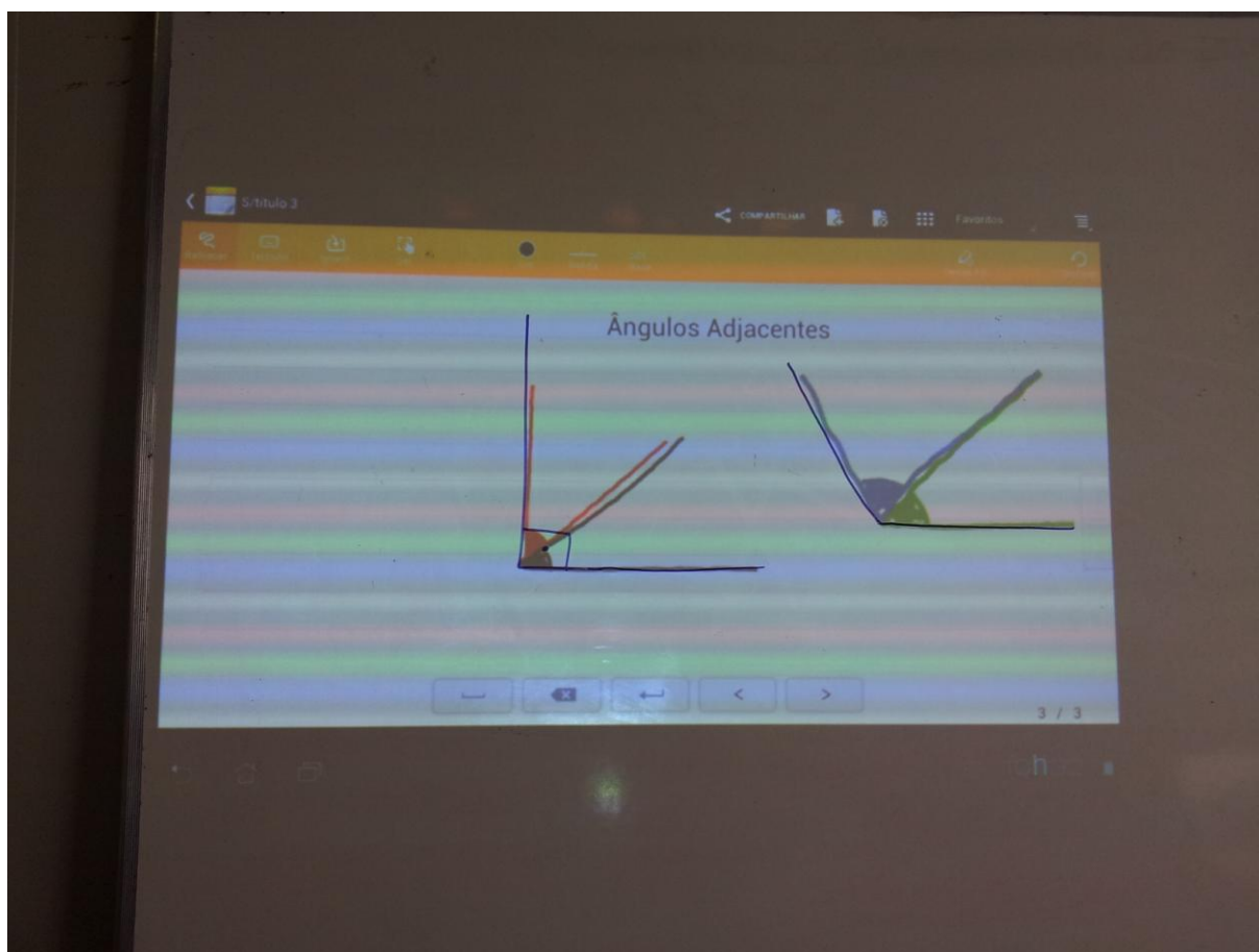
Figura 12: Ângulos Adjacentes
