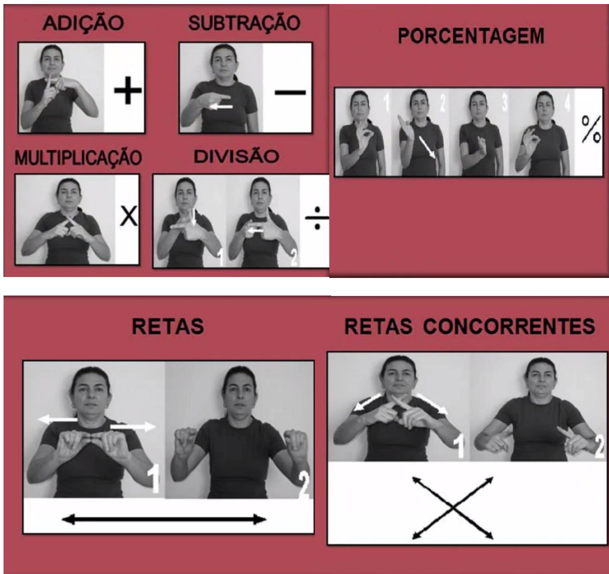
Figura 6: Sinais Matemáticos em LIBRAS
