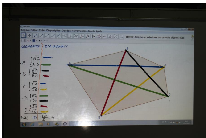
Figura 16: Diagonais do Pentágono
