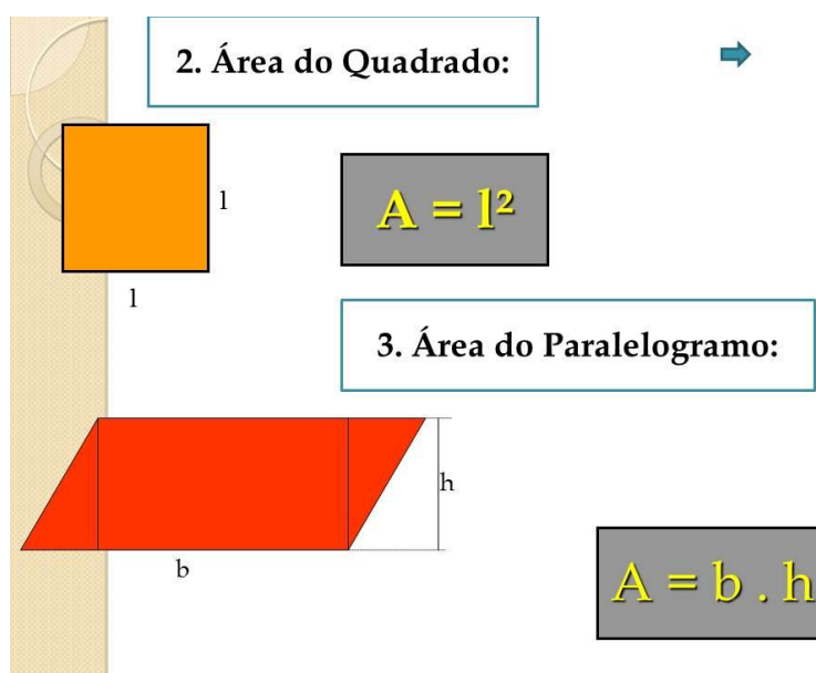
Figura 28: Formalizando as ideias sobre cálculos de áreas
