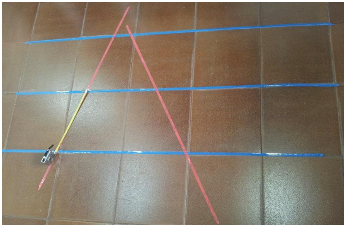
Figura 25: Aprendendo Teorema de Thales
