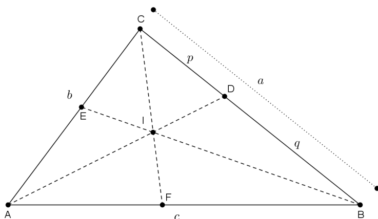
Figura 3.4: Triângulo e seu incentro
