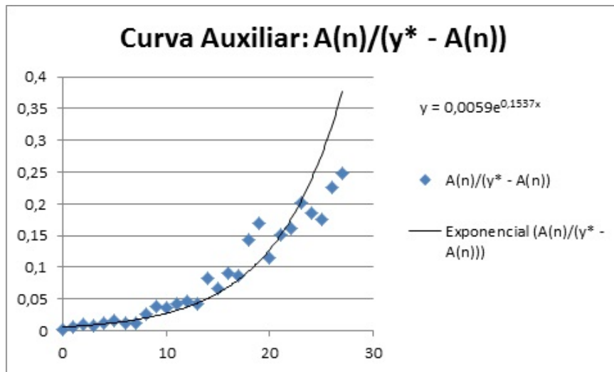
Figura 3.19: Curva auxiliar do modelo logístico 3
