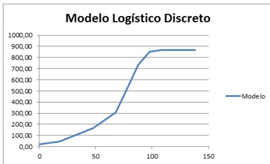
Figura 4.6: Curva do Modelo Logístico Discreto da população
