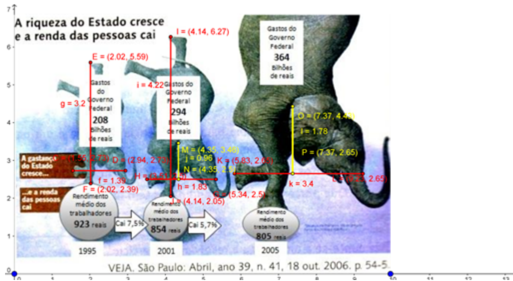
Figura 21 – A riqueza do estado cresce e a renda das pessoas cai mensurado no Geogebra.
