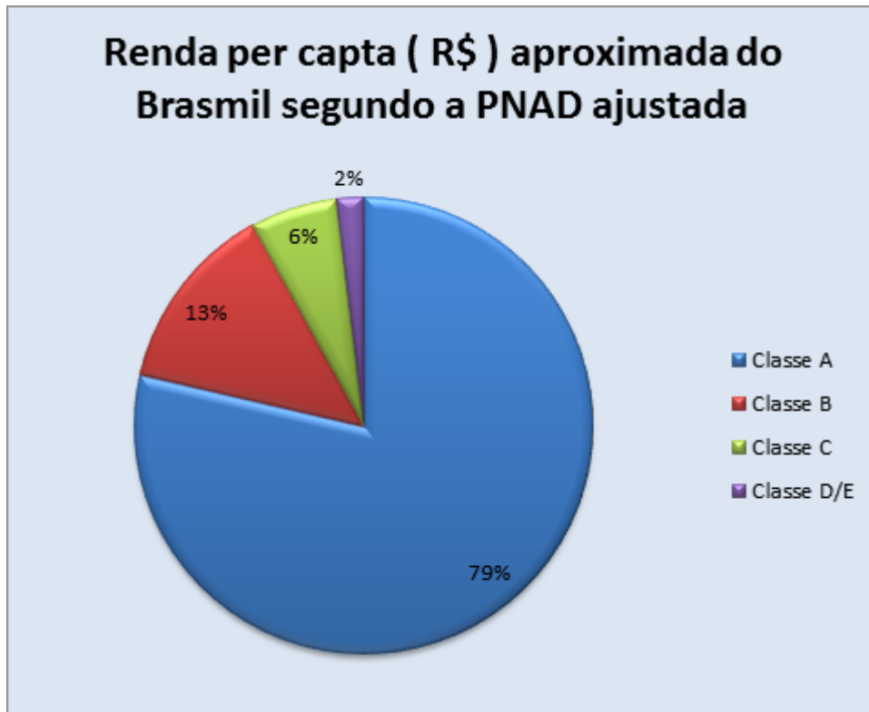
Figura 14 – Gráfico de setores comparativo da renda per capita, por classes no Brasmil.
