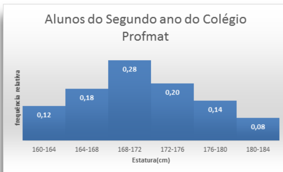
Figura 2 – Histograma relativo à estatura dos alunos do segundo ano do Colégio Profmat em frequência relativa.
