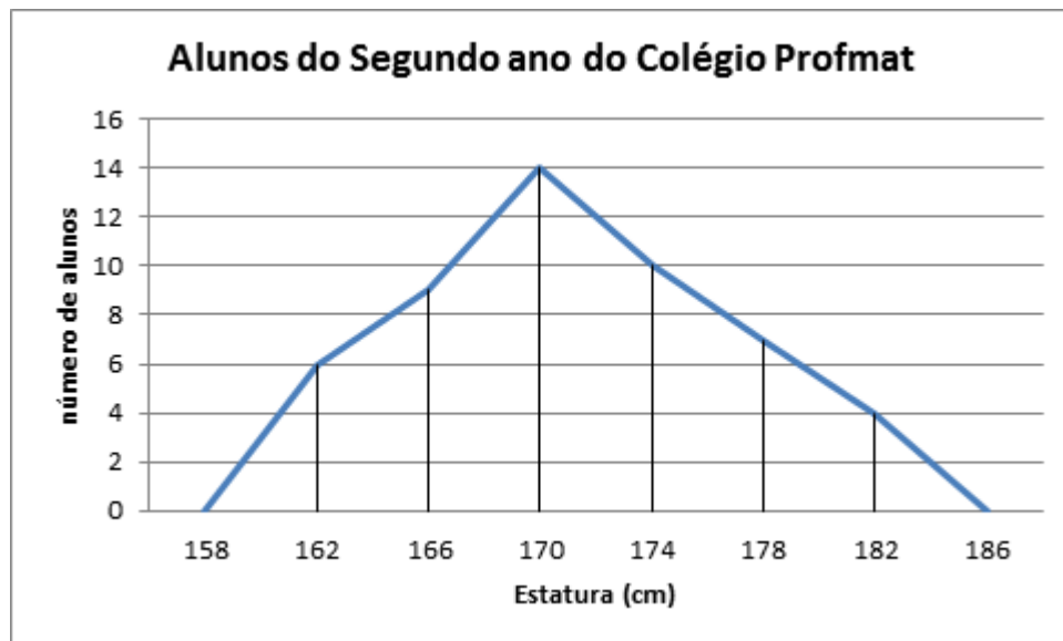
Figura 3 – Polígono de frequência relativo à estatura dos alunos do segundo ano do Colégio Profmat.
