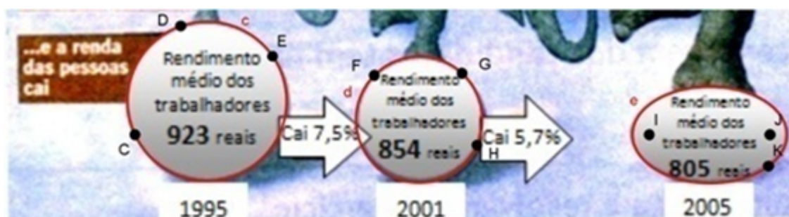
Figura 27 – Os círculos e a elipse.
