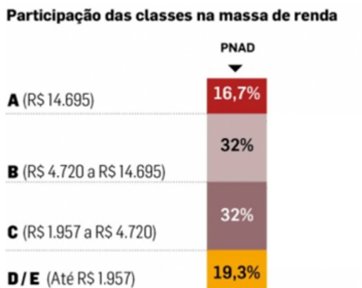
Figura 11 – Participação das classes na massa de renda segundo a PNAD.
