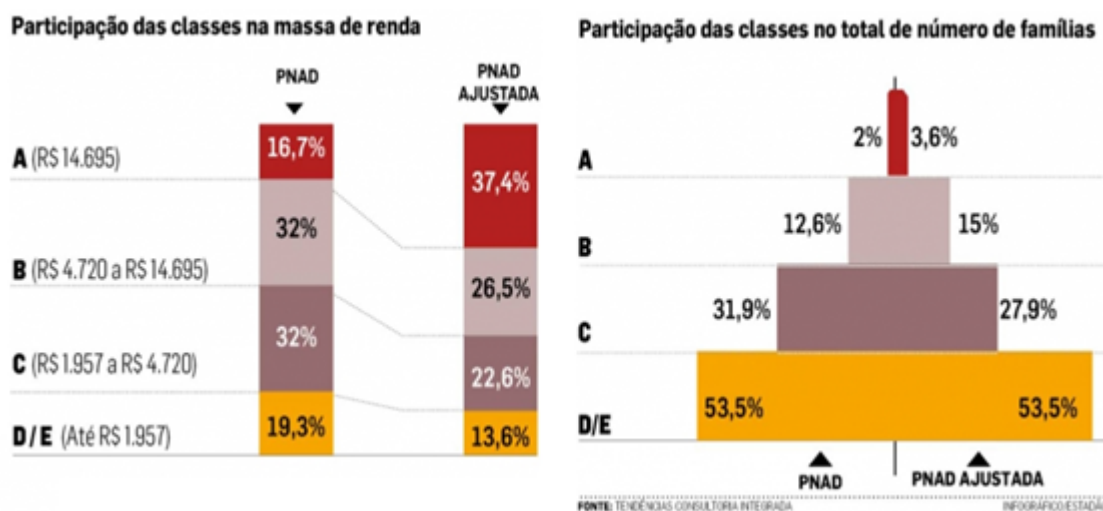
Figura 13 – Comparação da participação das classes na massa de renda segundo a PNAD e segundo a PNAD ajustada e comparação da participação das classes no total de número de famílias segundo a PNAD e segundo a PNAD ajustada.
