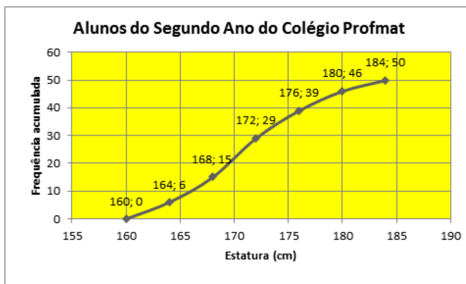
Figura 4 – Polígono de frequência acumulada relativo à estatura dos alunos do segundo ano do Colégio Profmat.
