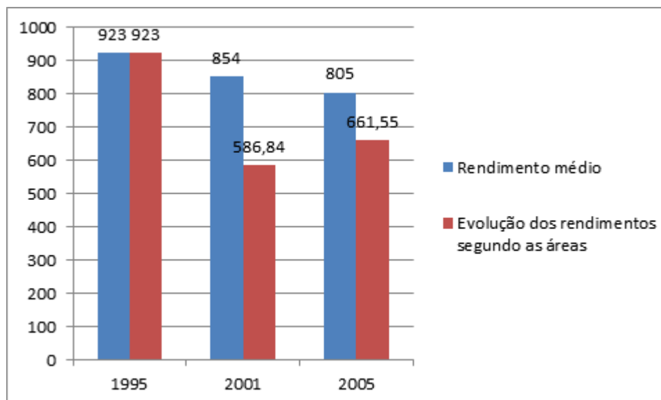
Figura 28 – rendimentos médios e rendimentos segundo as áreas.
