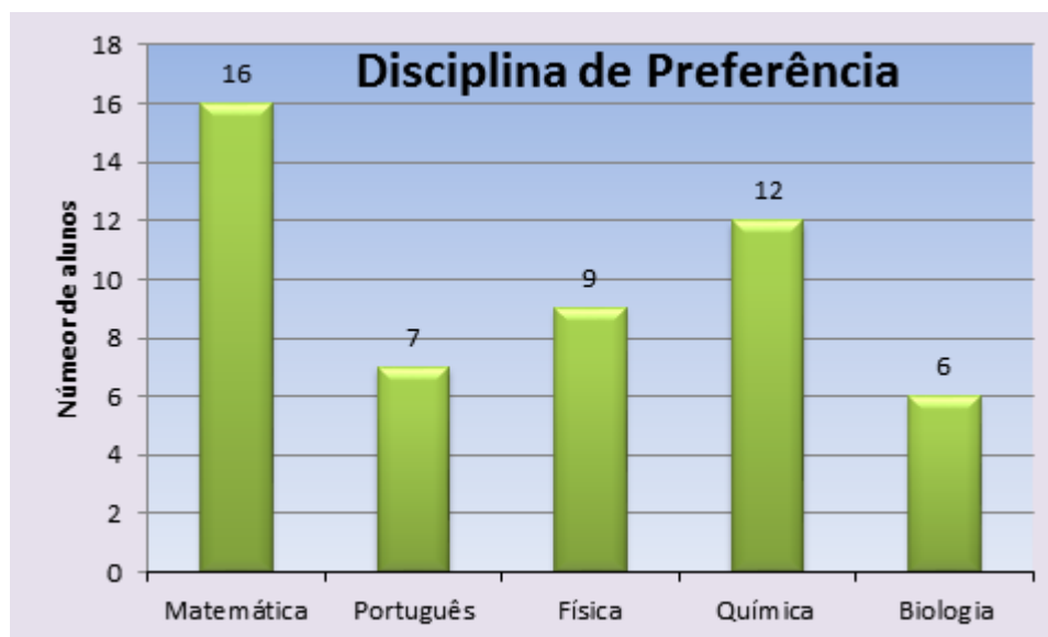
Figura 6 – Gráfico de barras relativo à disciplina de preferência.
