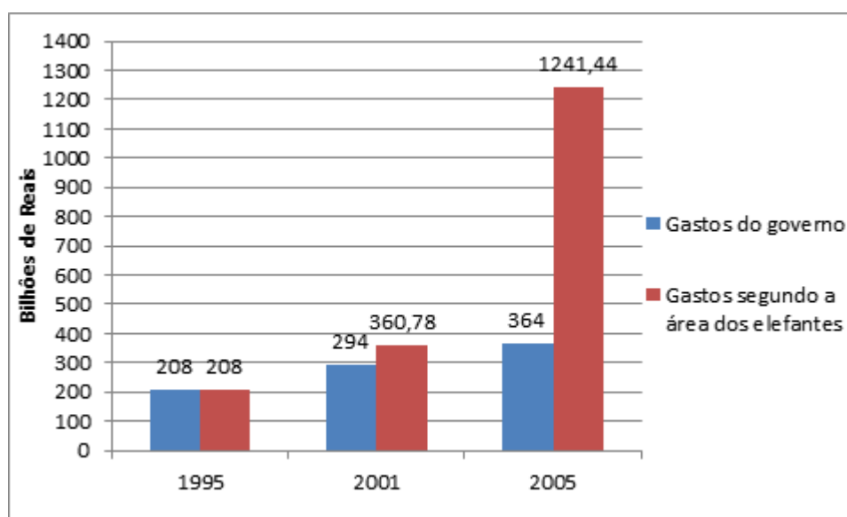
Figura 25 – Comparando os gastos do governo com suas respectivas representações gráficas.
