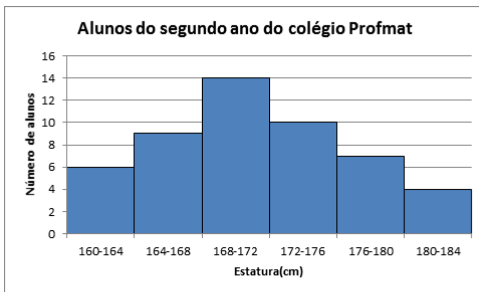
Figura 1 – Histograma relativo à estatura dos alunos do segundo ano do Colégio Profmat em números absolutos.
