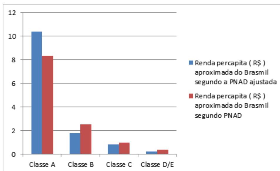
Figura 15 – Gráfico de barras comparativo das rendas per capita aproximadas do Brasmil, segundo a PNAD e do Brasmil, segundo a PNAD ajustada.
