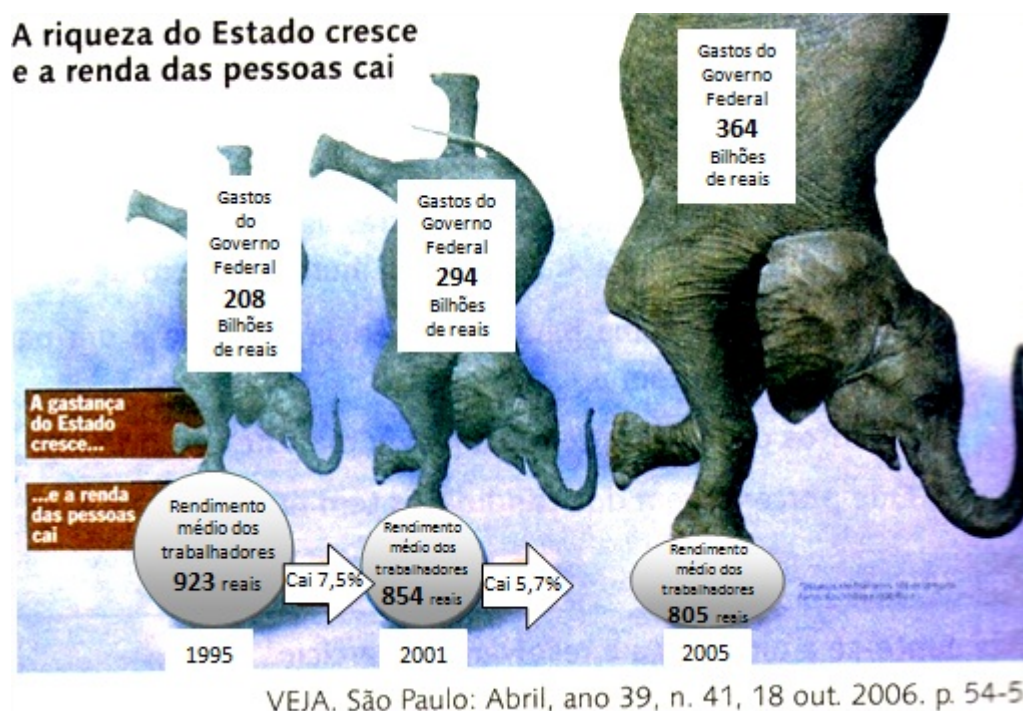
Figura 20 – A riqueza do estado cresce e a renda das pessoas cai.
