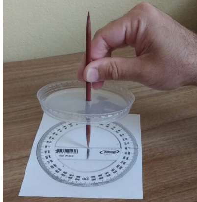
Figura 27 – Centralização da base do Teodolito
