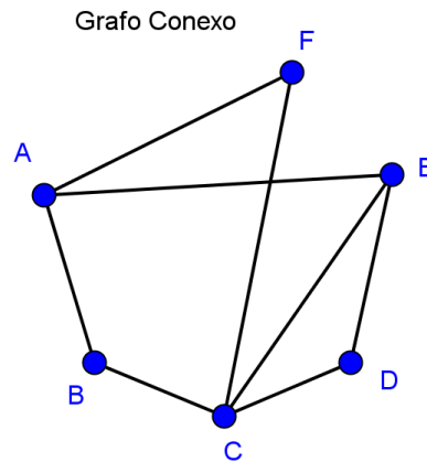
Figura 3.9: Grafo das relações de amizade.
