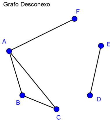
Figura 3.8: Grafo das relações familiares.
