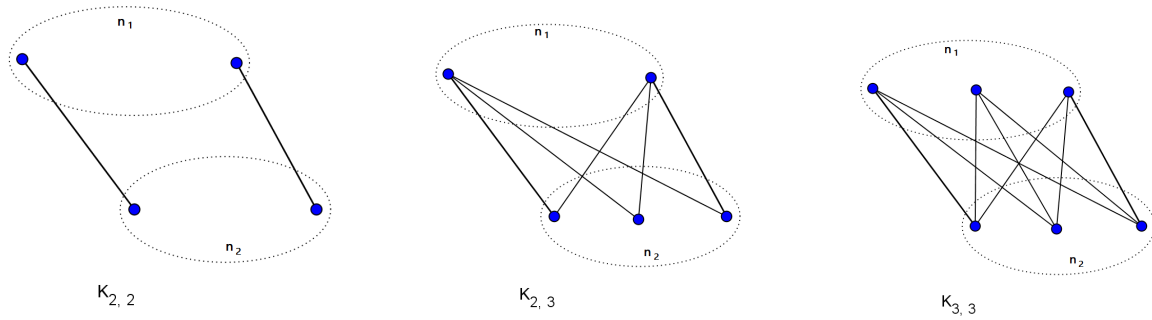
Figura 3.12: Grafos bipartidos K_{n_1, n_2} .
