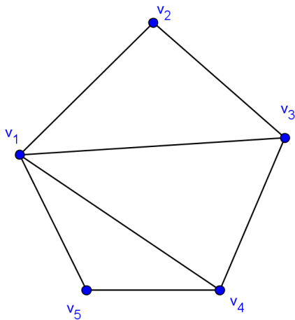
Figura 3.17: Grafo K_5 acrescido das arestas (v_1, v_3) e (v_1, v_4) .
