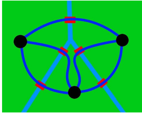
Figura 4.4: Grafo do problema da cidade de Barra do Corda.
