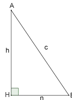
Figura 2.5: Triângulo retângulo em H e hipotenusa c
