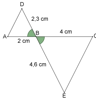
Figura 1.28: Triângulos
