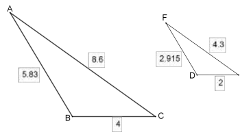
Figura 1.25: Triângulos
