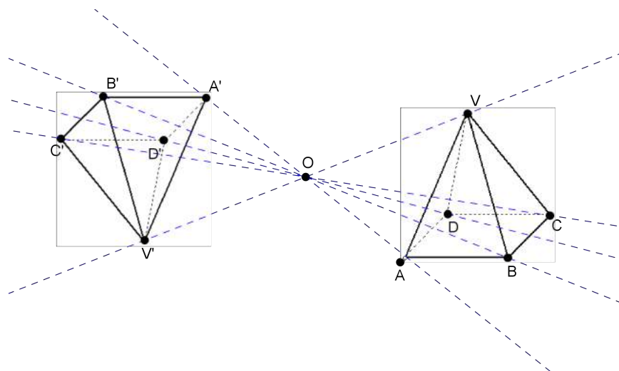
Figura 2.28: Pirâmide homotética
