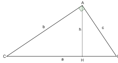
Figura 2.2: Triângulo retângulo com altura h
