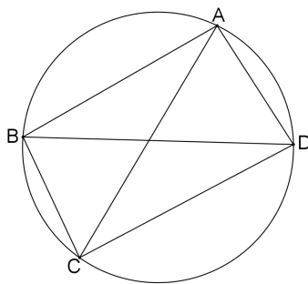
Figura 2.6: Quadrilátero inscrito
