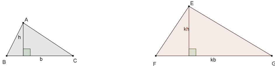
Figura 1.8: Triângulos de medidas proporcionais
