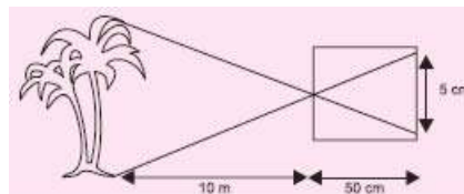
Figura 2.11: Árvore projetando imagem de 5 cm. Fonte: mundoeducacao.bol.uol.br
