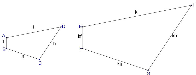
Figura 1.6: Quadriláteros semelhantes
