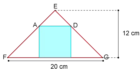
Figura 3.1: Quadrado inscrito em um triângulo
