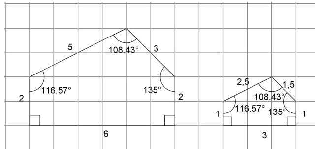
Figura 1.4: Polígonos semelhantes
