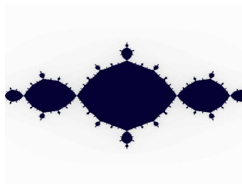
Figura 9: Conjunto de Julia ( c = -1 )
