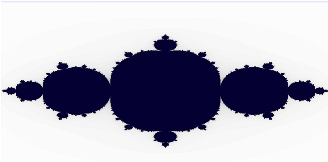
Figura 17: Conjunto de Julia ( c = -0.75 ) gerado pelo software ChaosPro
