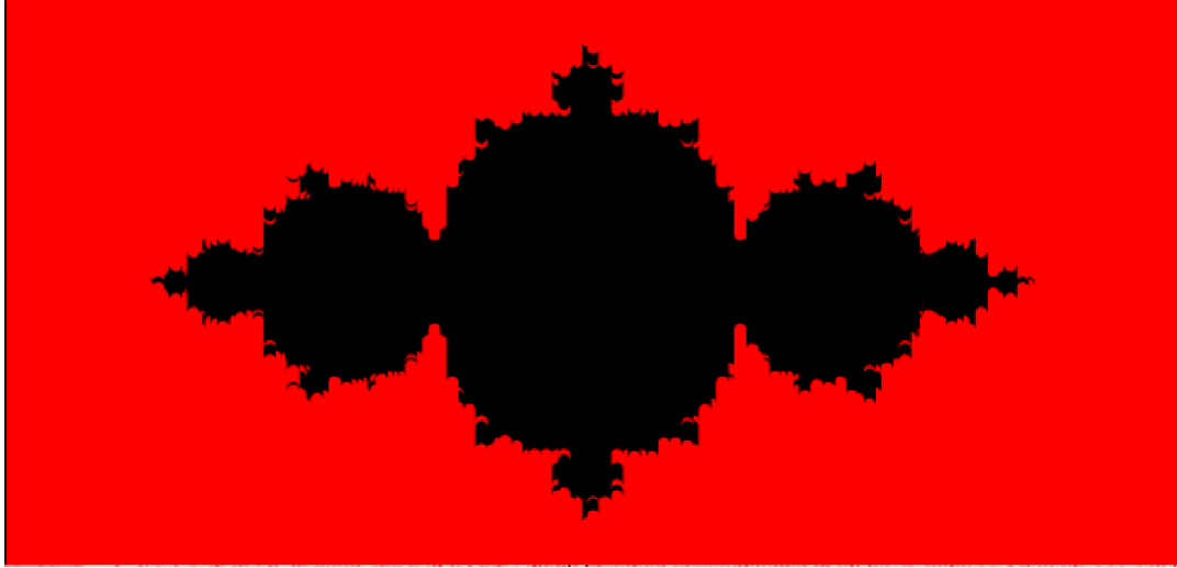
Figura 15: Conjunto de Julia ( c = -0.75 ) gerado pelo software Geogebra
