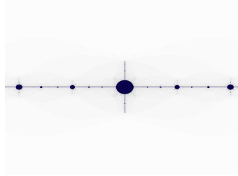
Figura 10: Conjunto de Julia (avião)
