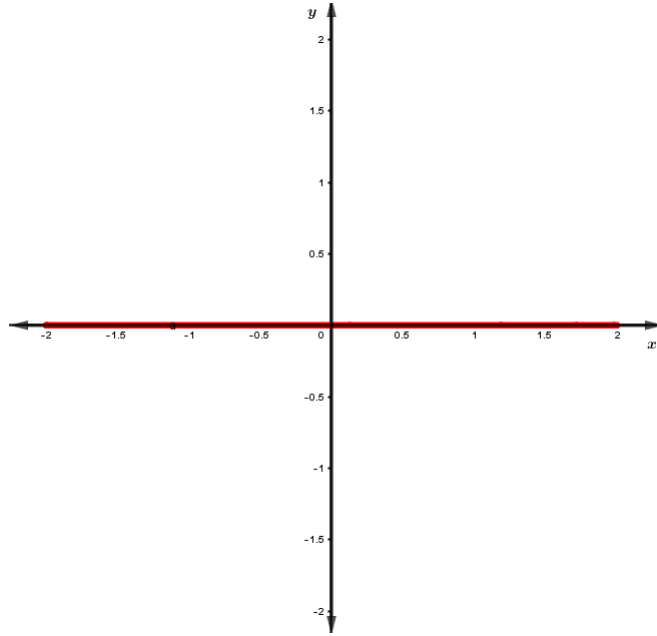
Figura 8: Conjunto de Julia ( c = -2 )
