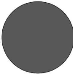
Figura 7: Conjunto de Julia preenchido ( c = 0 )
