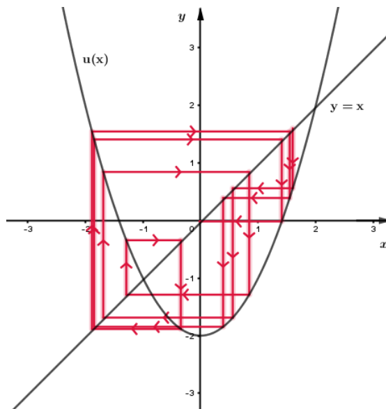
Figura 6: Iteração do ponto x_0 = 1.6
