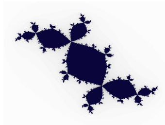
Figura 11: Conjunto de Julia (coelho)
