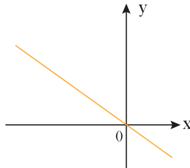
Figura 29-Representação da função do primeiro grau com raiz nula.
