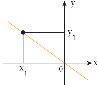
Figura 30-Construção do gráfico de uma função linear.
