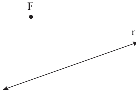
Figura 38-Reta no plano e um ponto fora dela.
