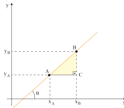
Figura 21-Triângulo retângulo com hipotenusa sobre a reta.
