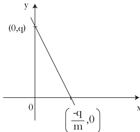
Figura 28-Representação gráfica da raiz da função do primeiro grau.
