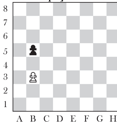
Figura 7-Localização de uma peça de xadrez por coluna e linha.
