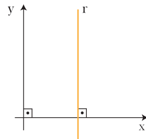
Figura 27-Reta vertical não representando uma função.
