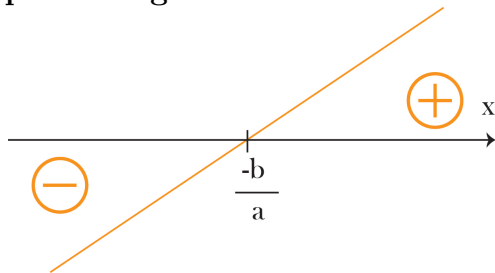
Figura 36-Estudo do sinal da função do primeiro grau crescente.
