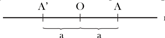
Figura 2-Distância de um ponto a origem.
