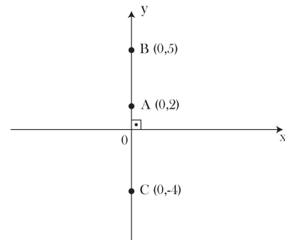
Figura 9-Ponto localizado sobre o eixo das ordenadas.
