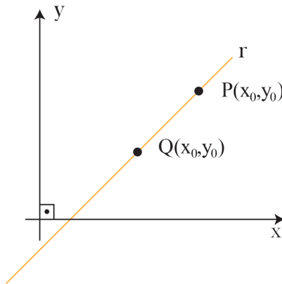
Figura 23-Ponto fixo e ponto genérico pertencentes a uma reta.
