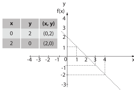
Figura 32- Gráfico de uma função do 1º grau decrescente.
