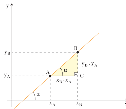
Figura 22-Triângulo retângulo para cálculo do coeficiente angular.
