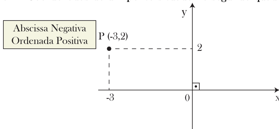
Figura 12-Coordenadas de um ponto situado no segundo quadrante.
