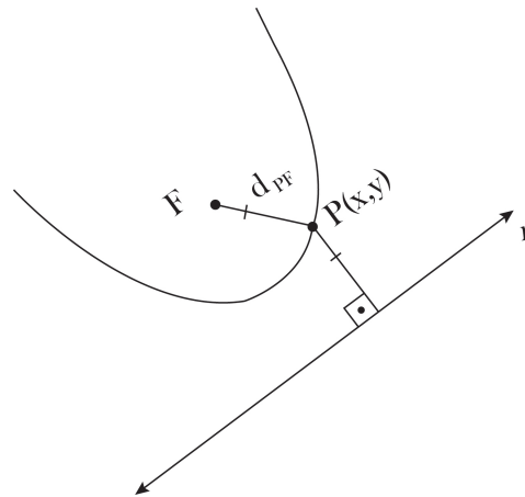
Figura 39-Determinação de uma parábola.
