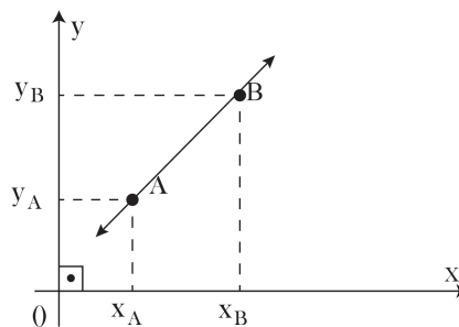
Figura 19-Representação de uma reta no plano cartesiano ortogonal.
