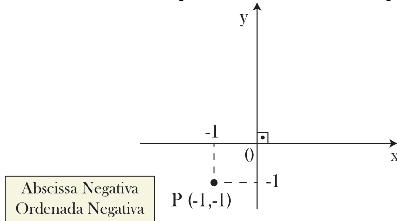
Figura 13-Coordenadas de um ponto situado no terceiro quadrante.
