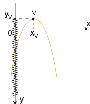
Figura 54-Imagem da função do segundo grau com concavidade para baixo
