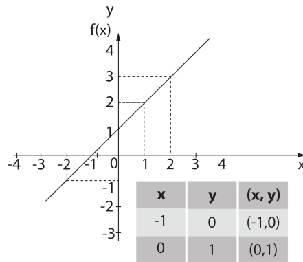
Figura 31-Gráfico de uma função do 1º grau crescente.
