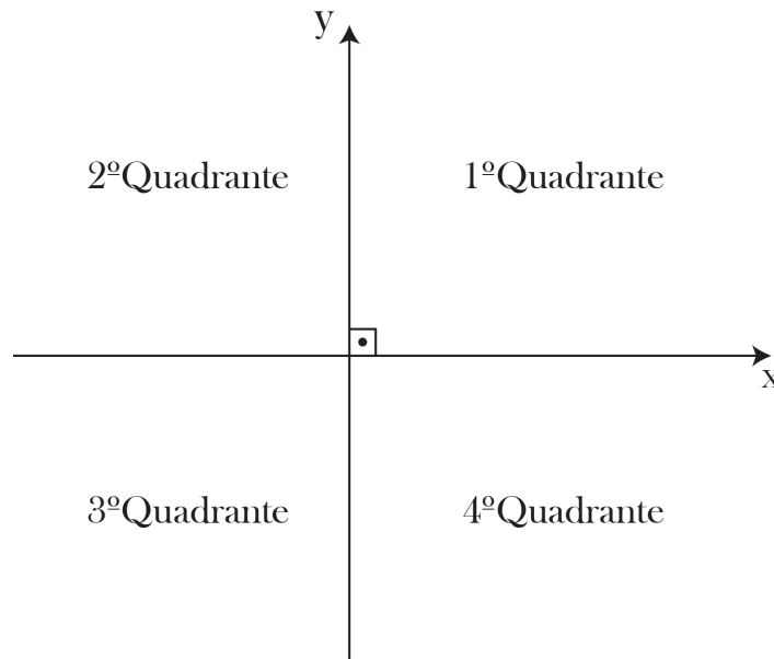
Figura 10-Posicionamento dos quadrantes no plano cartesiano ortogonal.
