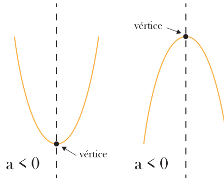
Figura 52-Máximo ou mínimo da função do segundo grau.
