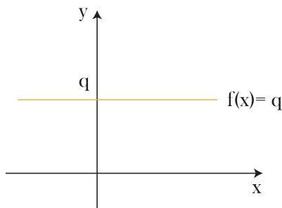
Figura 26-Reta horizontal determinando uma função constante.
