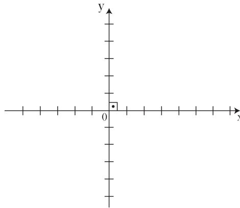
Figura 5-O plano cartesiano ortogonal.
