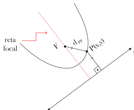
Figura 40-Reta focal de uma parábola.
