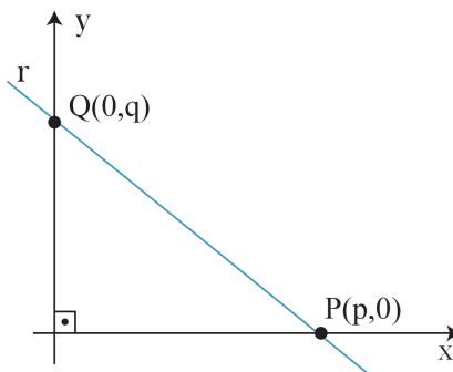
Figura 25-Intersecção da reta com o eixo das abscissas e das ordenadas.
