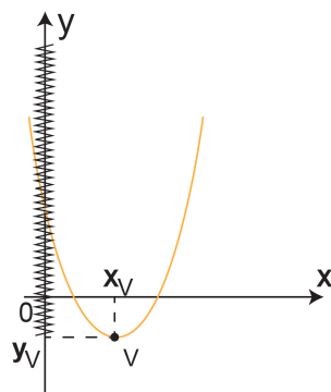
Figura 53-Imagem da função do segundo grau com concavidade para cima.
