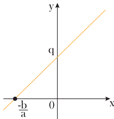
Figura 33- Reta com coeficiente angular e termo independente positivos.
