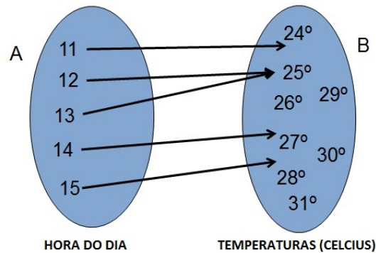
Figura 16-Domínio e Contradomínio da função representada em diagrama.
