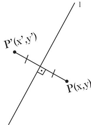
Figura 41-Simetria com relação ao eixo focal.
