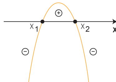
Figura 56-Sinal da imagem da função do segundo grau com a < 0 e \Delta > 0 .
