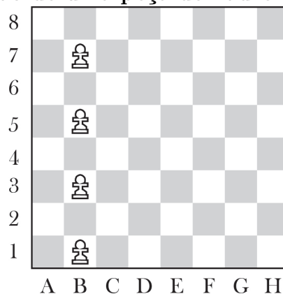
Figura 4-Localização de uma peça de xadrez apenas por coluna.
