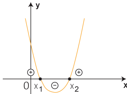
Figura 55-Sinal da imagem da função do segundo grau com a > 0 e \Delta > 0 .
