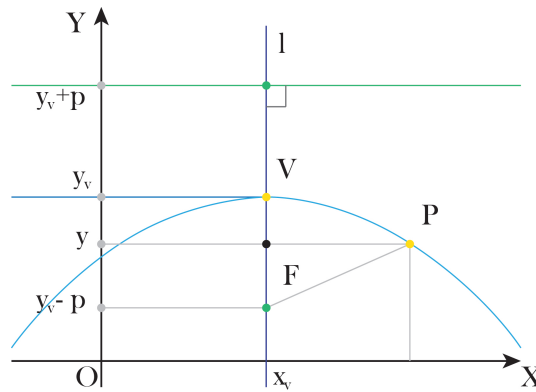
Figura 48-Parábola com concavidade para baixo e vértice fora da origem.
