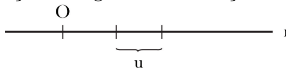
Figura 1-Localização da origem e determinação da unidade na reta.
