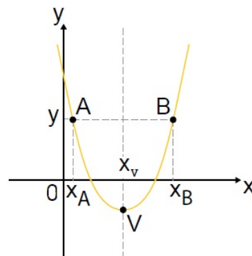
Figura 44-Relação entre pontos com abscissas equidistantes da abscissa do vértice.
