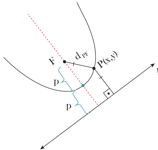
Figura 43-Representação gráfica do parâmetro da parábola.
