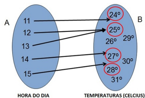
Figura 17-Imagem da função representada em diagrama.
