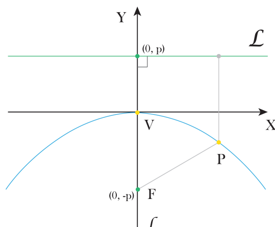
Figura 46-Parábola com foco abaixo da origem e vértice na origem.
