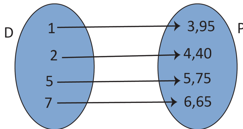
Figura 15-Representação de uma relação no diagrama de flechas.
