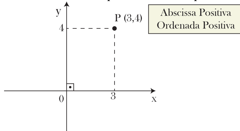
Figura 11-Coordenadas de um ponto situado no primeiro quadrante.
