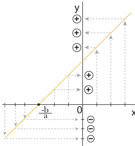
Figura 34-Relação entre valores da abscissa e o sinal da imagem da função do primeiro grau.
