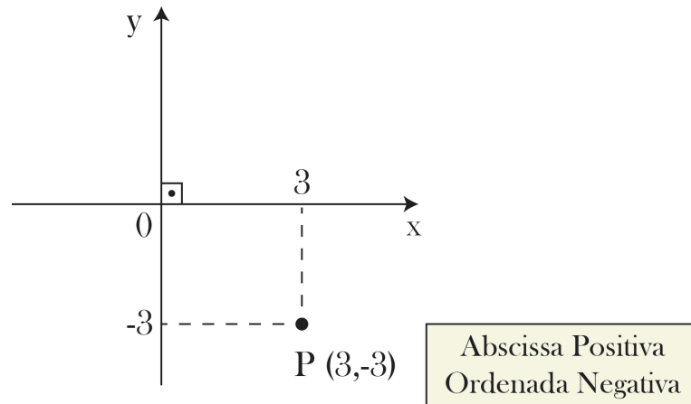
Figura 14-Coordenadas de um ponto situado no quarto quadrante.
