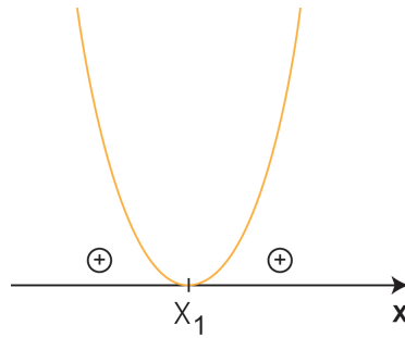
Figura 57-Sinal da imagem da função do segundo grau com a > 0 e \Delta = 0 .
