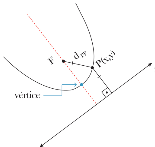
Figura 42-Vértice de uma parábola.
