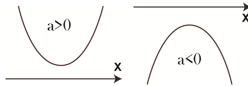
Figura 51-Função do segundo grau sem raízes reais.
