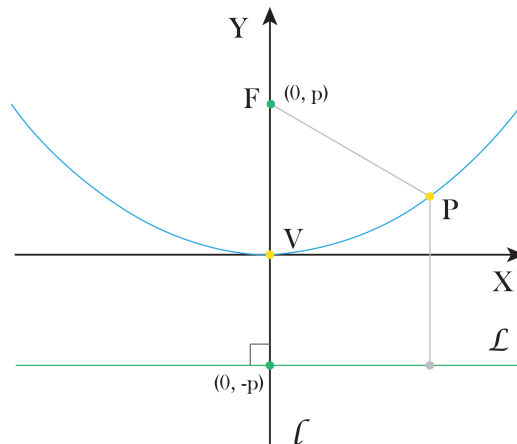
Figura 45-Parábola com foco acima da origem e vértice na origem.
