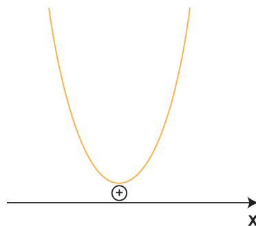
Figura 59-Sinal da imagem da função do segundo grau com a > 0 e \Delta < 0 .
