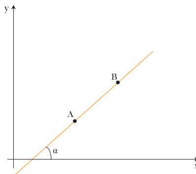
Figura 20-Ângulo formado entre uma reta e o eixo das abscissas.
