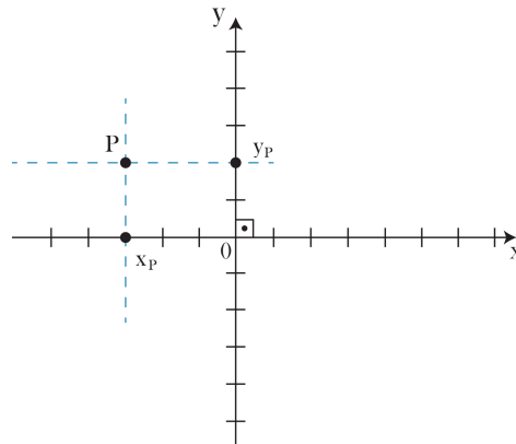
Figura 6-Projeções ortogonais de um ponto no plano cartesiano.
