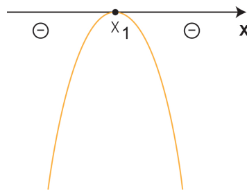
Figura 58-Sinal da imagem da função do segundo grau com a < 0 e \Delta = 0 .
