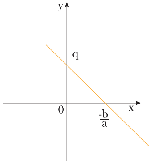
Figura 35-Reta com coeficiente angular negativo e termo independente positivo.
