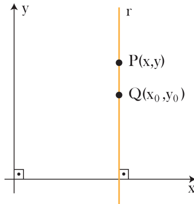
Figura 24-Reta paralela ao eixo das ordenadas.
