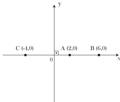
Figura 8-Ponto localizado sobre o eixo das abscissas.
