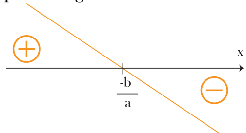
Figura 37-Estudo do sinal da função do primeiro grau decrescente.
