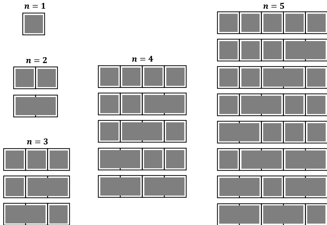
Figura 21 – Contagem dos possíveis modos de cobertura de uma malha 1 \times n , para n \leq 5
