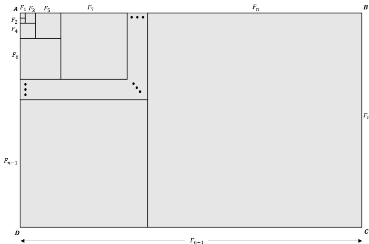
Figura 24 – Expansão da Figura 23 até o quadrado de lado F_n
