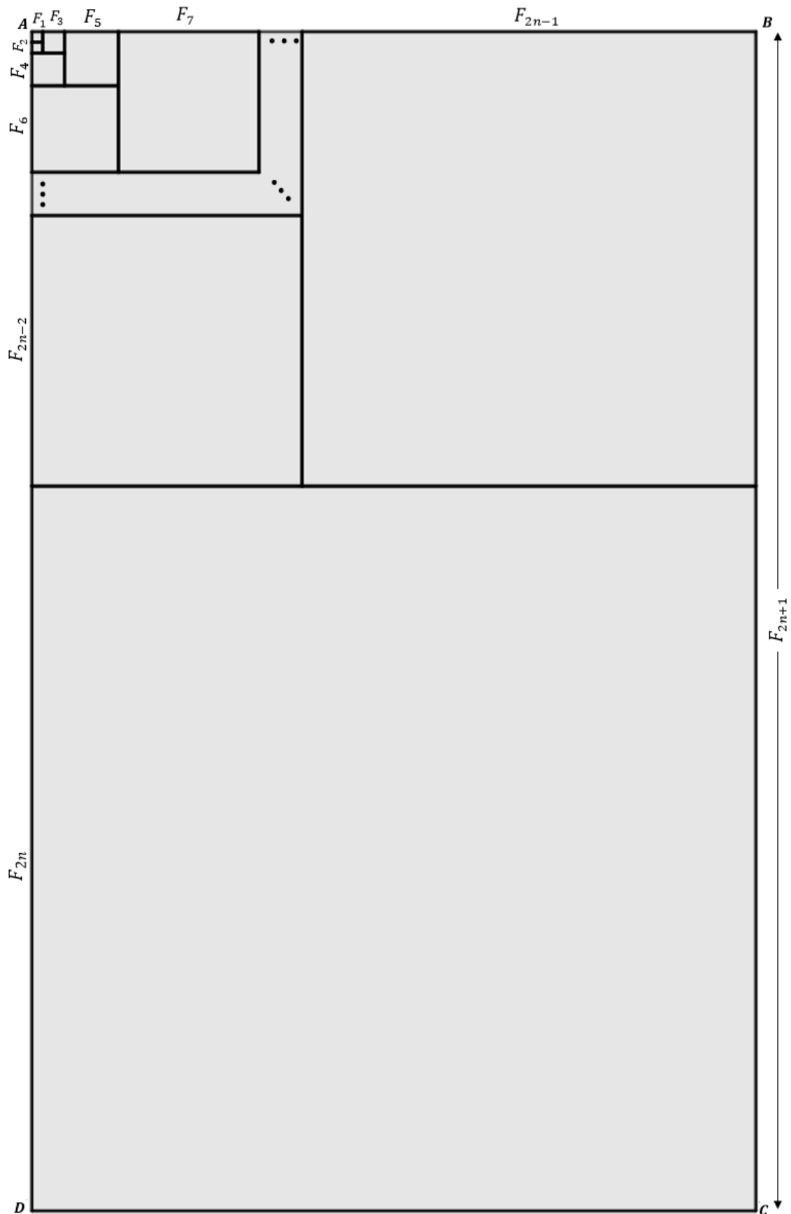
Figura 25 – Expansão da Figura 23 até o quadrado de lado F_{2n}
