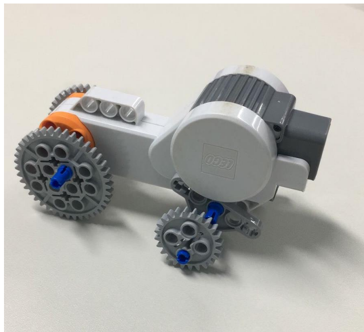
Figura 3- ENGRENAGENS
