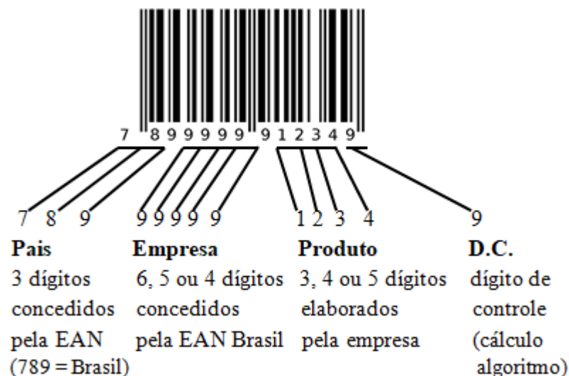
Figura 2 – Código EAN13
