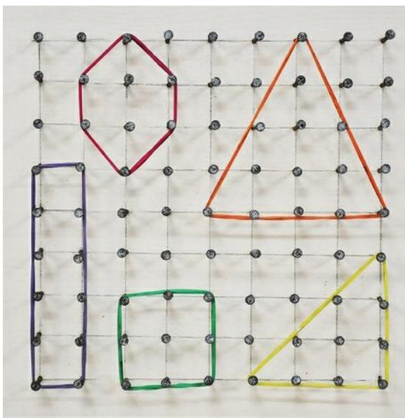
Figura 03 - Geoplano.
