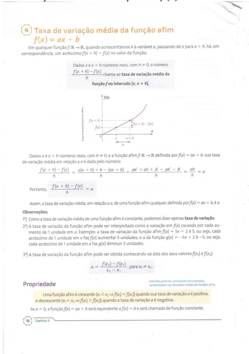
Figura 2 – Taxa de variação média de uma função afim f(x) = ax + b
