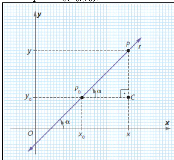
Figura 16 - Reta r contendo um ponto P_0(x_0, y_0) , de coordenadas conhecidas
