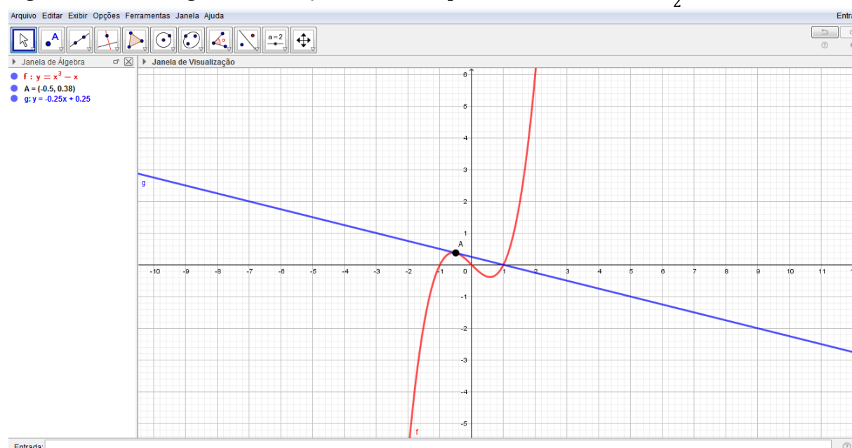
Figura 57 - Reta tangente à curva y = x^3 - x no ponto de abscissa x = -\frac{1}{2}
