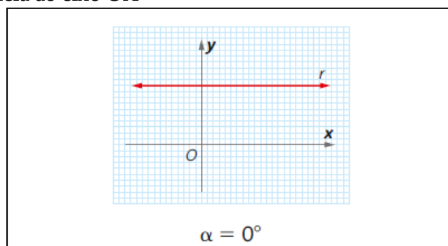
Figura 13 - Reta paralela ao eixo OX
