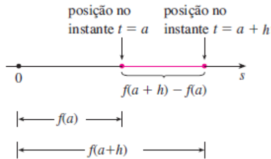
Figura 27 - Variação da posição de um objeto sobre uma reta r
