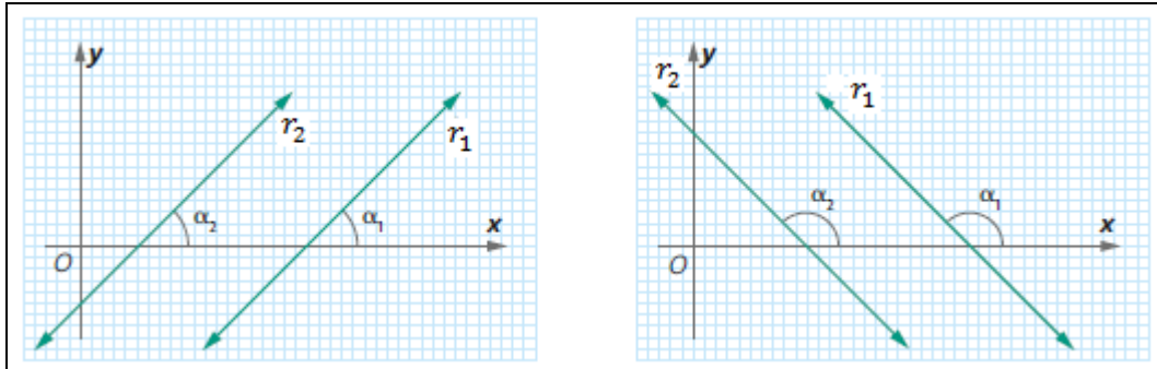
Figura 18 - Retas paralelas de inclinação \alpha_1 e \alpha_2
