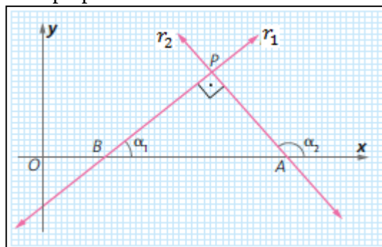
Figura 20 - Retas concorrentes perpendiculares
