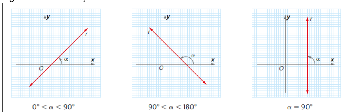
Figura 12 - Retas não paralelas ao eixo OX
