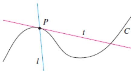
Figura 21 - Exemplos de retas tangentes a uma curva
