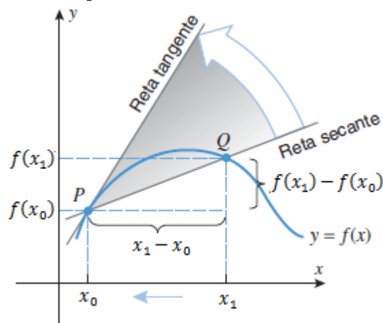
Figura 23 - Aproximação de Q e P pela direita
