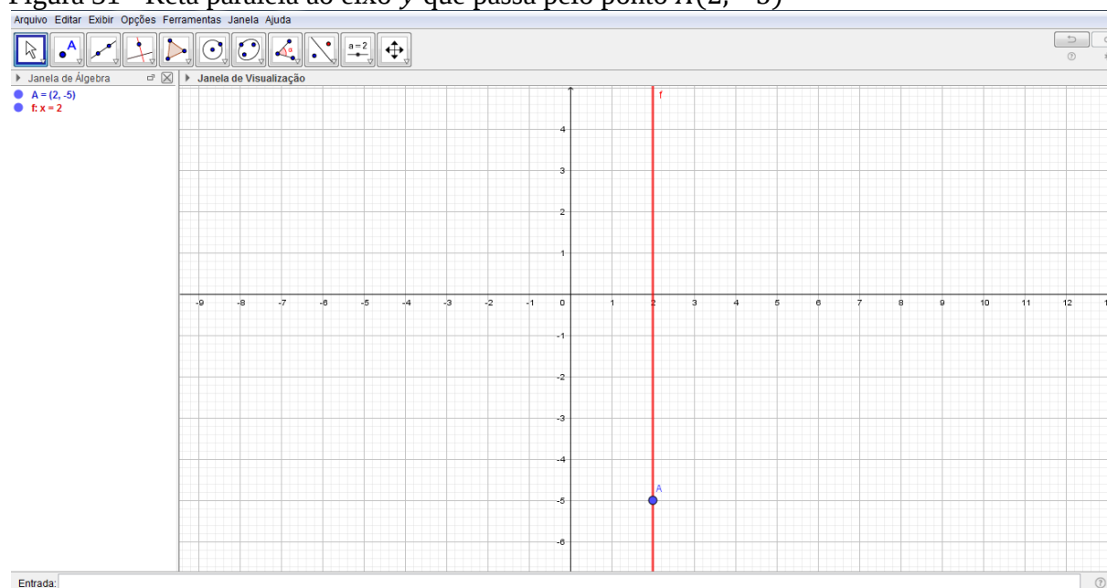
Figura 31 - Reta paralela ao eixo y que passa pelo ponto A(2, -5)
