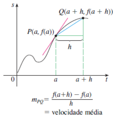
Figura 28 - Variação da posição de um objeto sobre a reta secante \overrightarrow{PQ}
