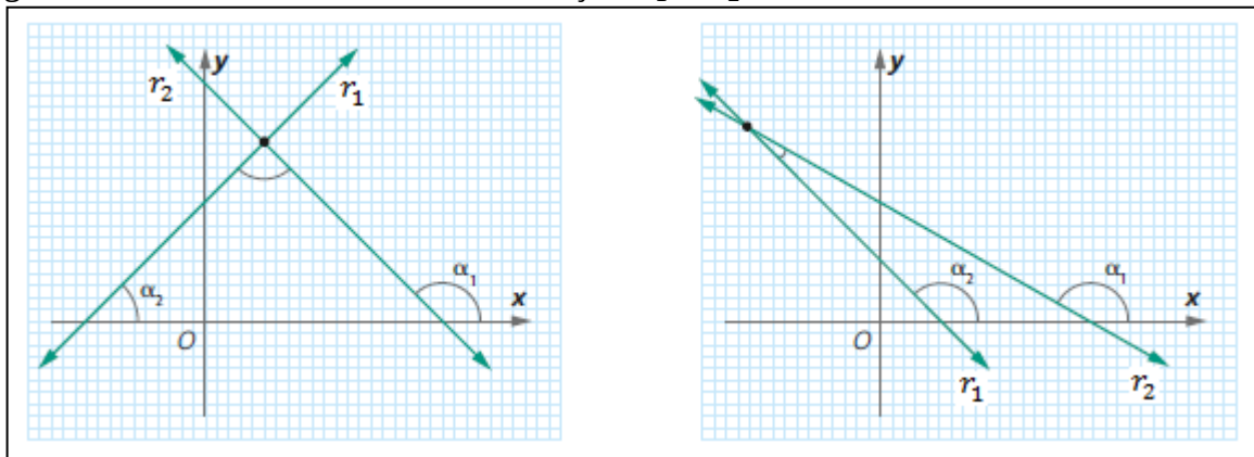
Figura 19 - Retas concorrentes com inclinação \alpha_1 e \alpha_2
