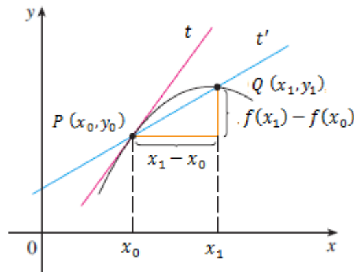
Figura 22 - Reta tangente t e reta secante t'
