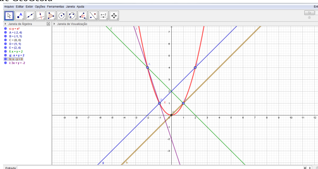
Figura 30 - Gráfico da função f(x) = x^2 com algumas retas secantes apresentado no software GeoGebra
