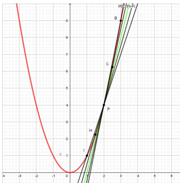
Figura 42 - Determinação da reta tangente a parábola y = x^2 por meio de aproximações de retas secantes
