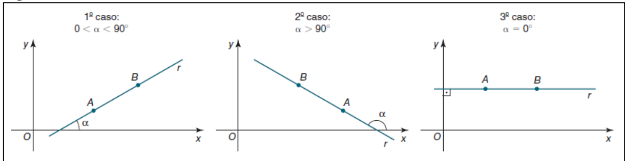
Figura 14 - Pontos distintos A e B sobre a reta r
