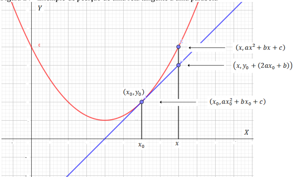
Figura 24 - Exemplo de posição de uma reta tangente a uma parábola
