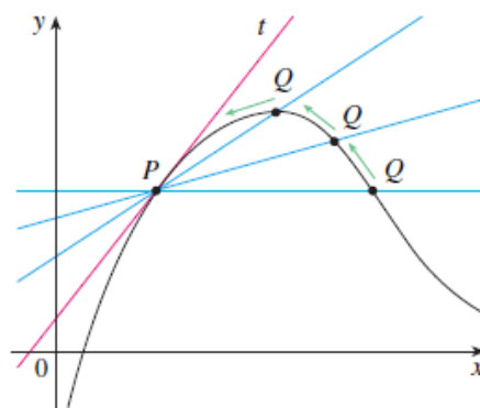
Figura 25 - Aproximação da reta secante \overline{PQ} à tangente t
