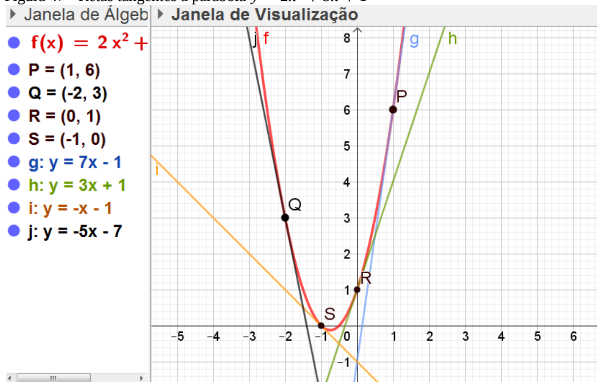
Figura 47 - Retas tangentes à parábola y = 2x^2 + 3x + 1
