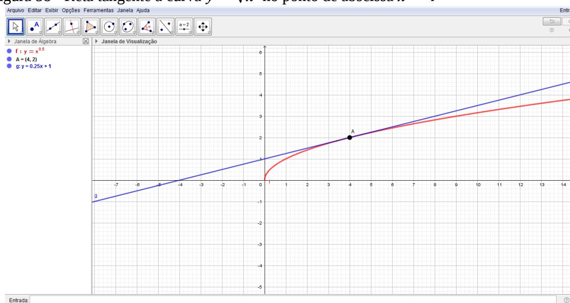
Figura 58 - Reta tangente à curva y = \sqrt{x} no ponto de abscissa x = 4
