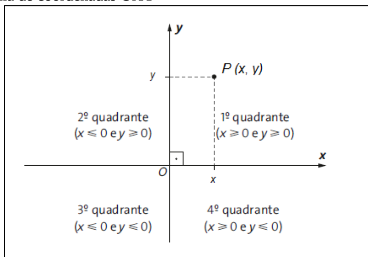
Figura 11 - Sistema de coordenadas OXY
