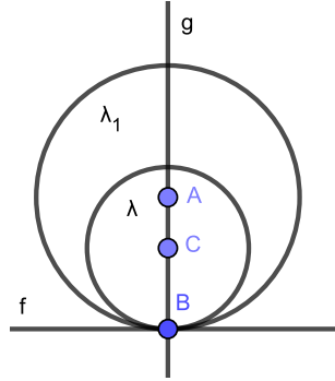
Figura 11: Tangentes internas.
