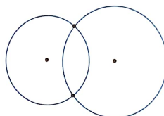
secantes
