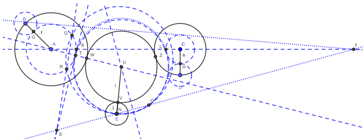
Figura 70: Três circunferências.
