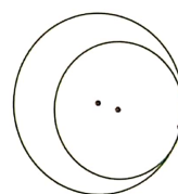
tangentes interiormente
