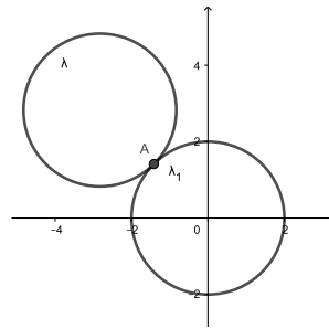
Figura 2: Representação geométrica.
