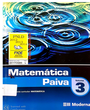
Figura 25: Matemática Paiva.
