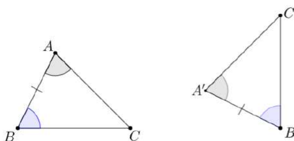
Figura 17 – Caso de congruência: ALA
