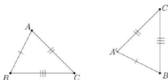
Figura 18 – Caso de congruência: LLL
