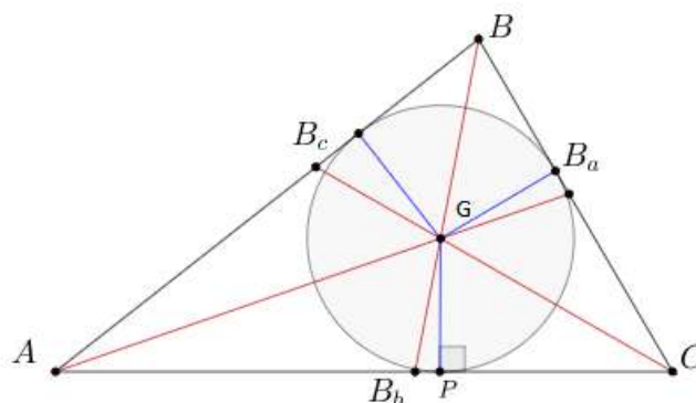
Figura 49 – O incentro
