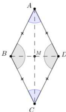
Figura 13 – Losango
