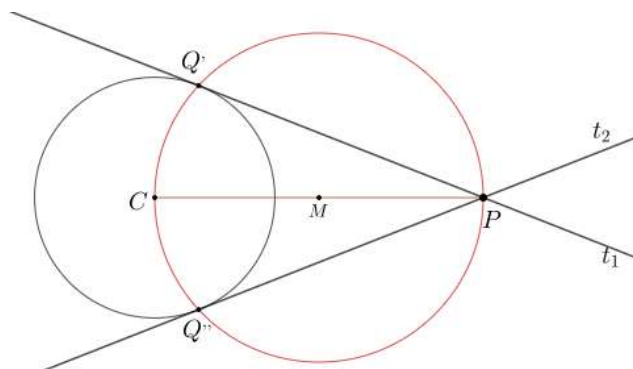
Figura 52 – O círculo, um ponto e suas tangentes
