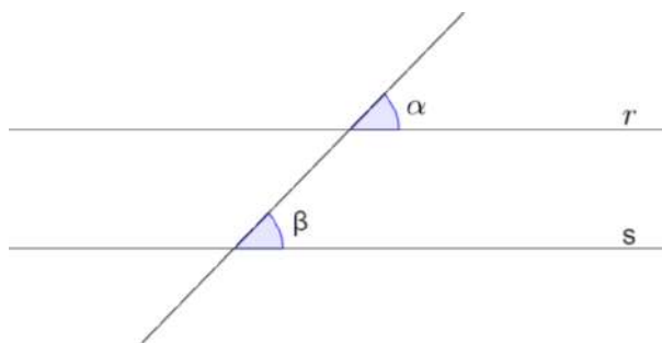
Figura 10 – Retas paralelas cortadas por uma transversal
