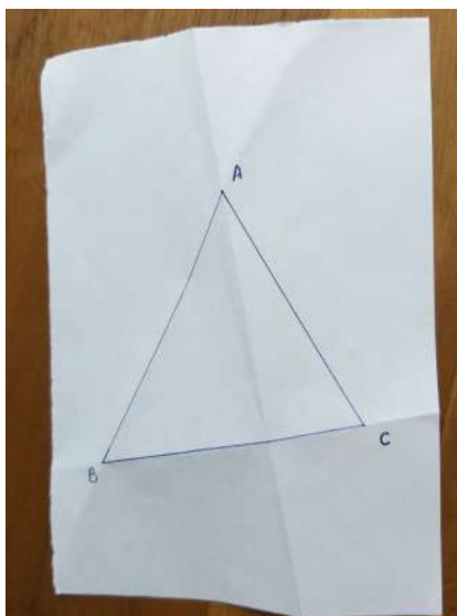
Figura 93 – Construção do ortocentro - passo 2
