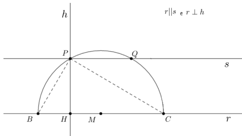
Figura 58 – Triângulo retângulo \triangle BPC
