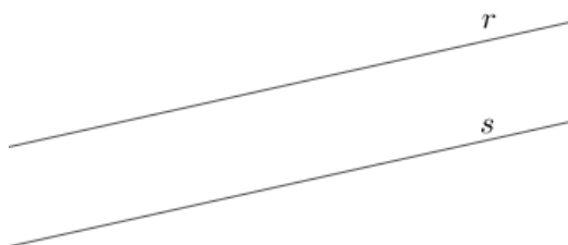
Figura 8 – Retas paralelas
