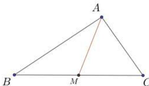
Figura 23 – A mediana
