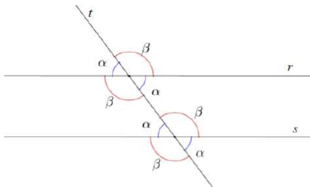
Figura 9 – Retas paralelas cortadas por uma transversal
