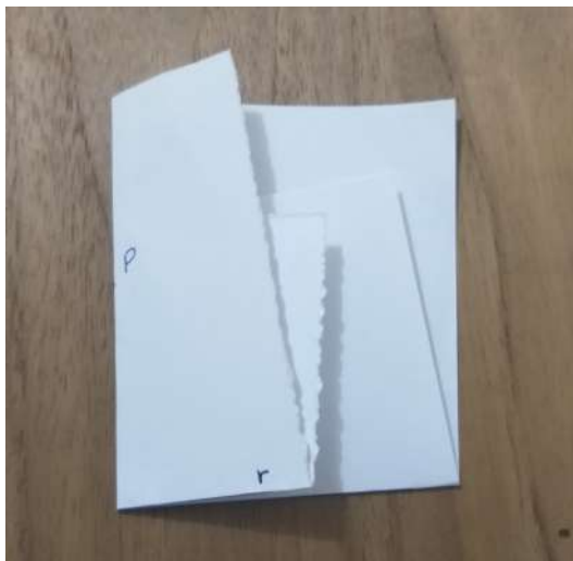
Figura 72 – Construção da uma reta perpendicular - passo 2
