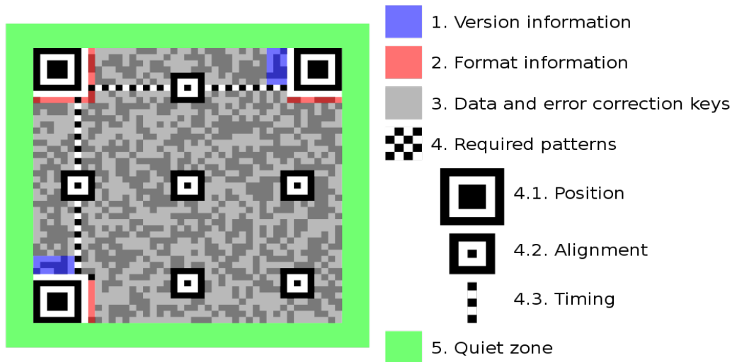
Figura 3: Estrutura do QR Code
