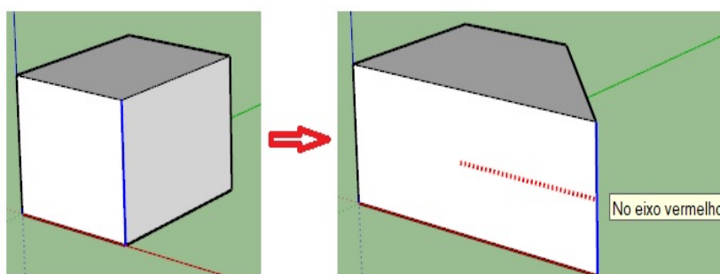
Figura 30 – Ferramenta “Mover”.
