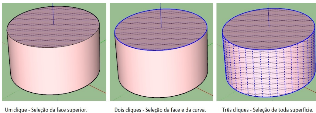
Figura 23 – Ferramenta “Selecionar”.
