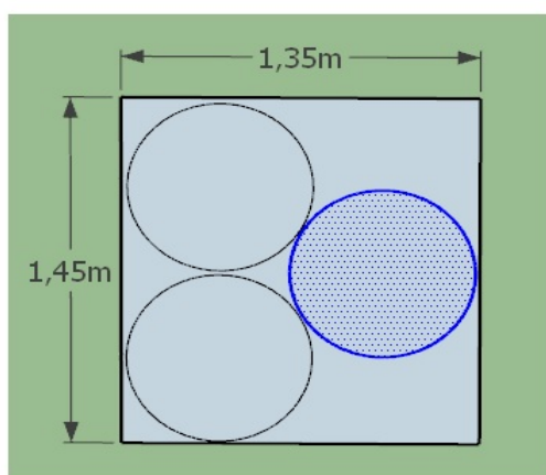
Figura 91 – Atividade 5 – Tarefa 4.
