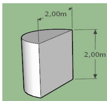
Figura 40 – Ferramenta “Dimensões”.
