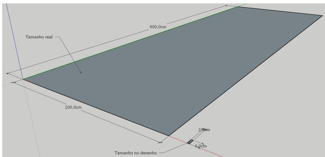
Figura 67 – Atividade 2 – Tarefa 4.
