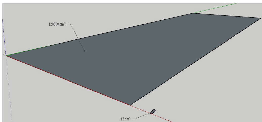
Figura 68 – Atividade 2 – Tarefa 5.
