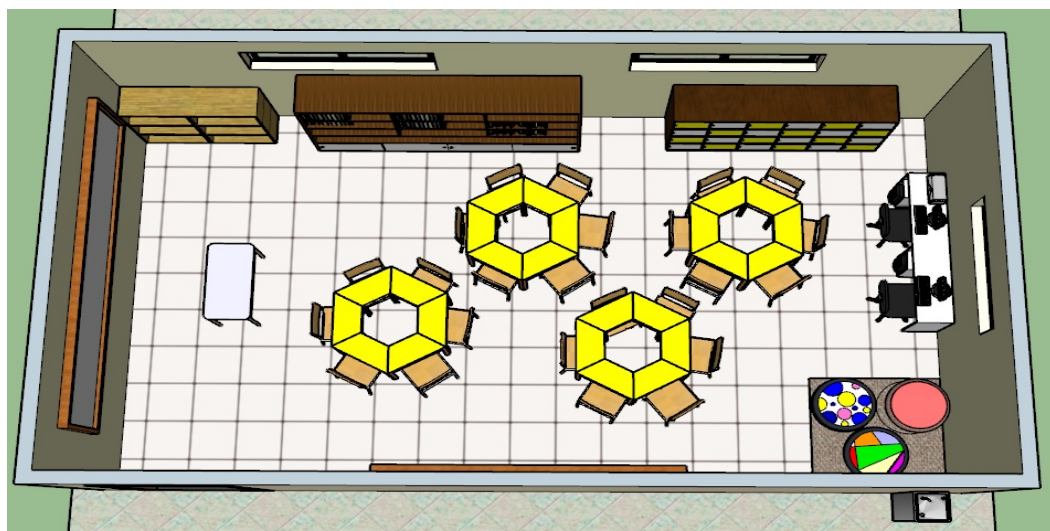
Figura 106 – Atividade 5 - Tarefa 22.
