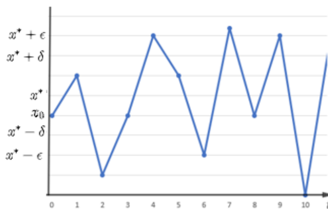
Figura 13. x^* instável
