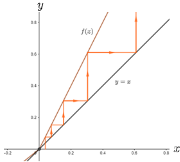
Figura 15. x^* = 0 é instável
