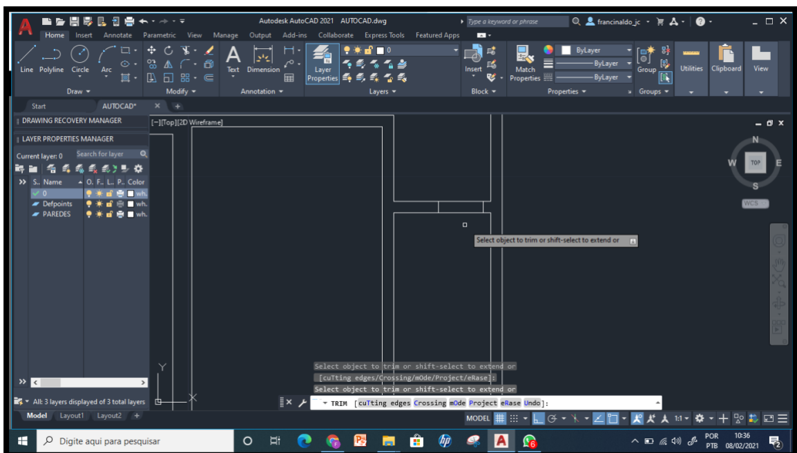
Figura 32: Construção das portas: banheiro (60cm) e as demais (80cm)
