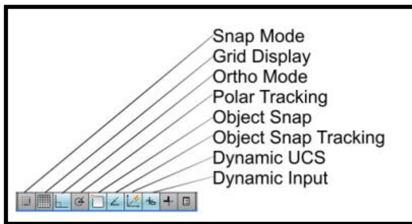
Figura 14: Barra de Rodapé do Autocad
