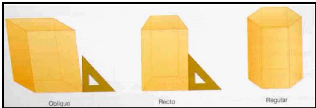
Figura 8: Classificação do Prisma e a definição do Paralelepípedo reto-retângulo
