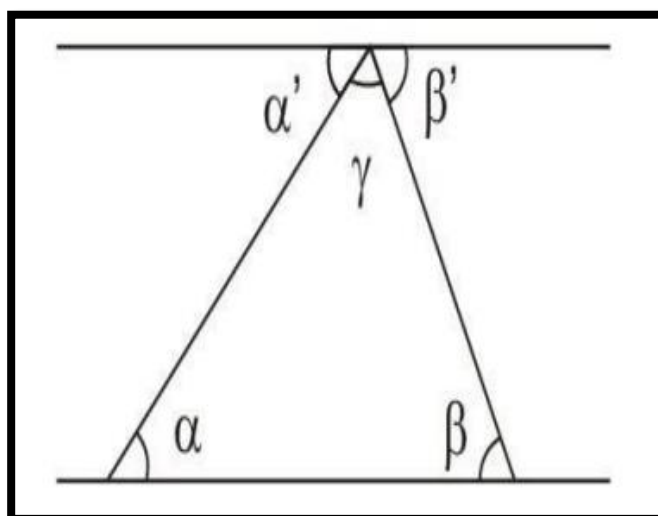
Figura 7: Princípios Básicos de Geometria Plana
