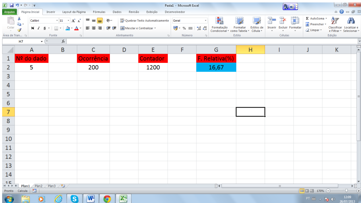
Figura 6.4: simulação do problema da seção 4.1
