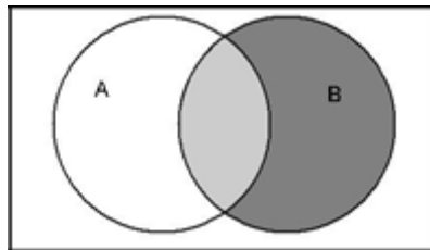
Figura 3.4: diagrama de venn para a proposição 3 da seção 3.3
