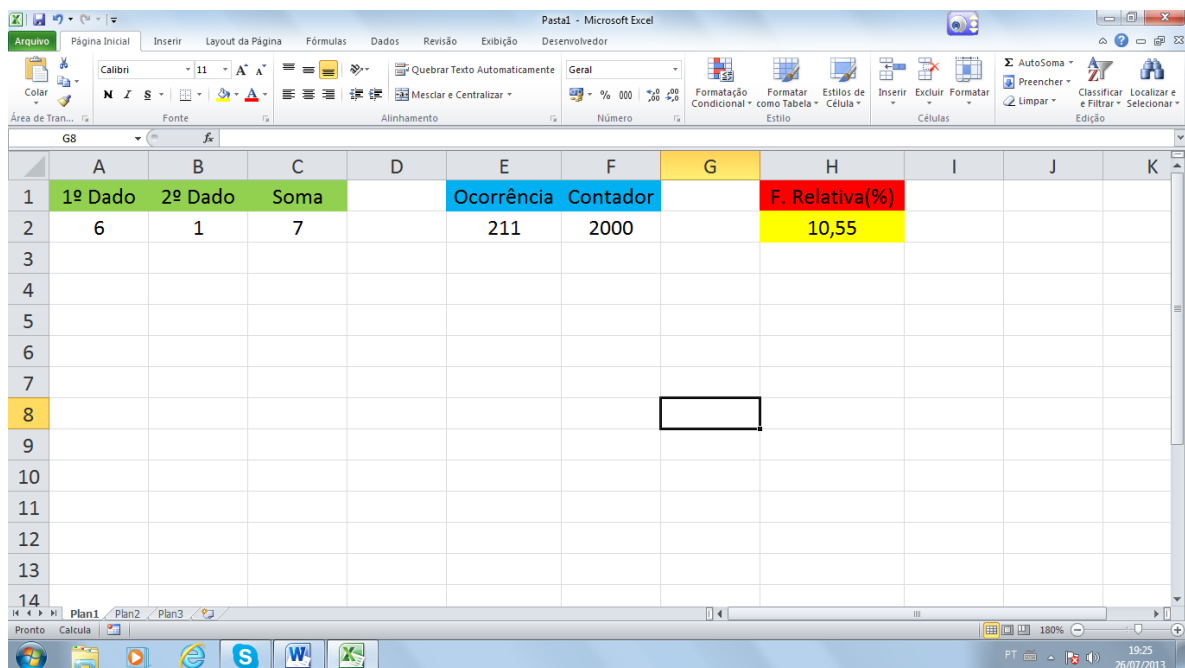
Figura 6.5: simulação do problema da seção 4.2
