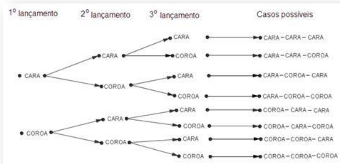
Figura 3.1: diagrama de árvores
