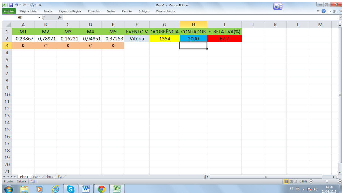
Figura 6.7: simulação do problema da seção 4.3
