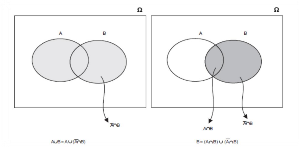
Figura 3.3: diagramas de venn para a proposição 2 da seção 3.3
