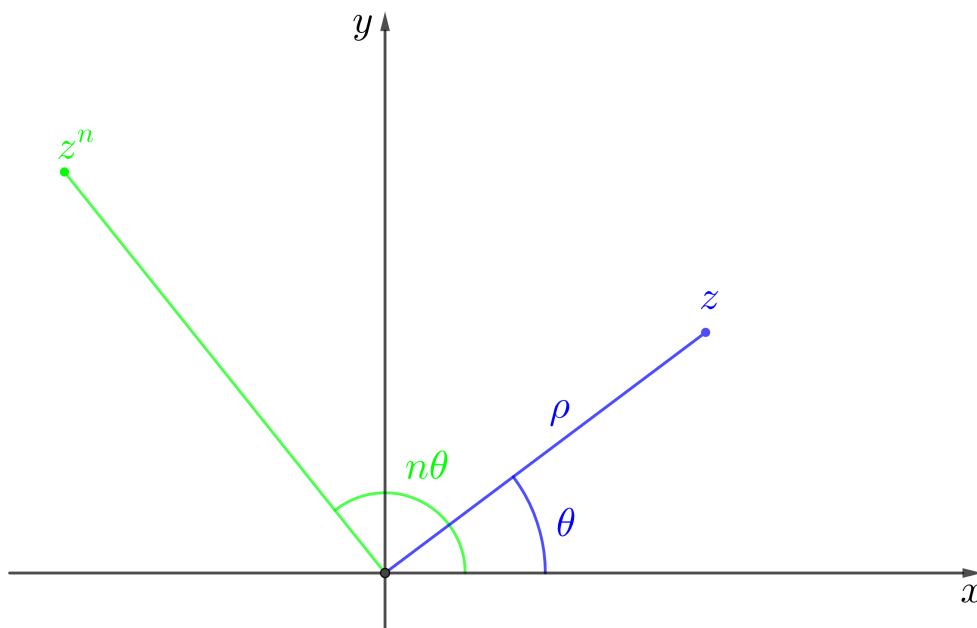
Figura 5 – Apresentação polar de z e z^n para o caso \rho > 1 e n > 1 .
