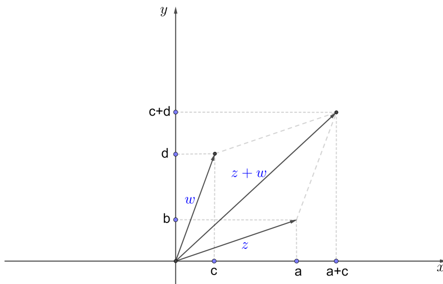
Figura 3 – Representação geométrica de z, w e z + w no \mathbb{R}^2
