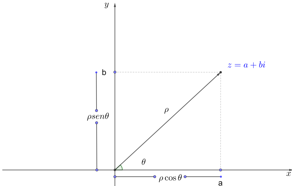
Figura 4 – Apresentação polar de z
