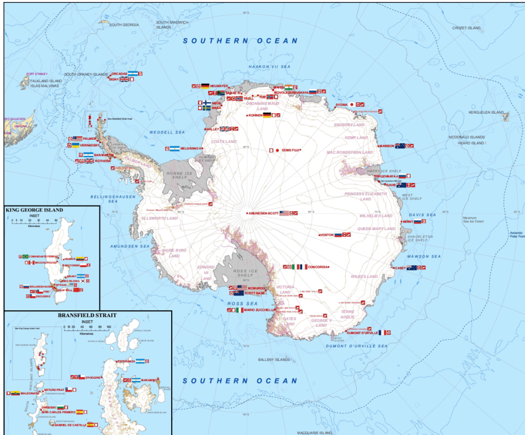
Figura 8 – Exemplo de Projeção Estereográfica do Pólo Sul
