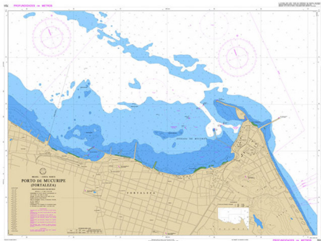
Figura 10 – Exemplo de Projeção de Mercator do Porto do Mucuripe (Fortaleza-CE)
