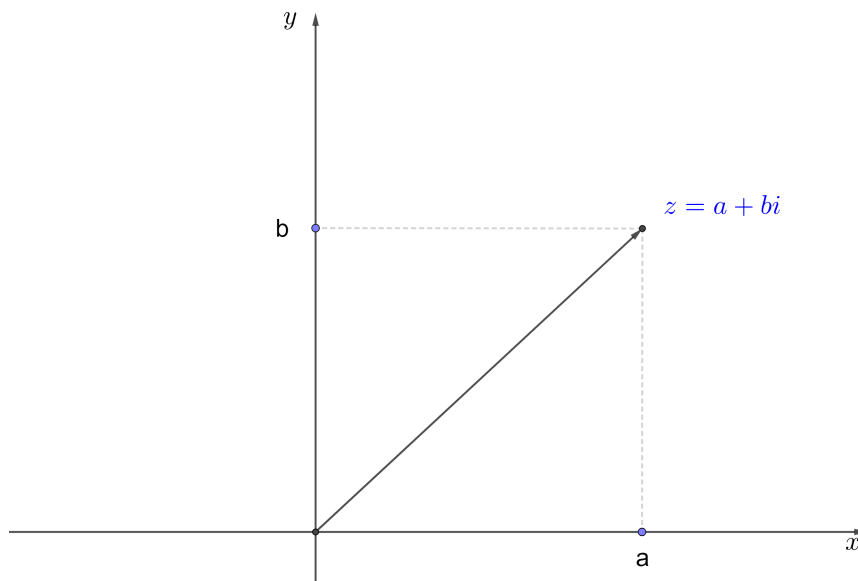
Figura 2 – Plano de Argand-Gauss
