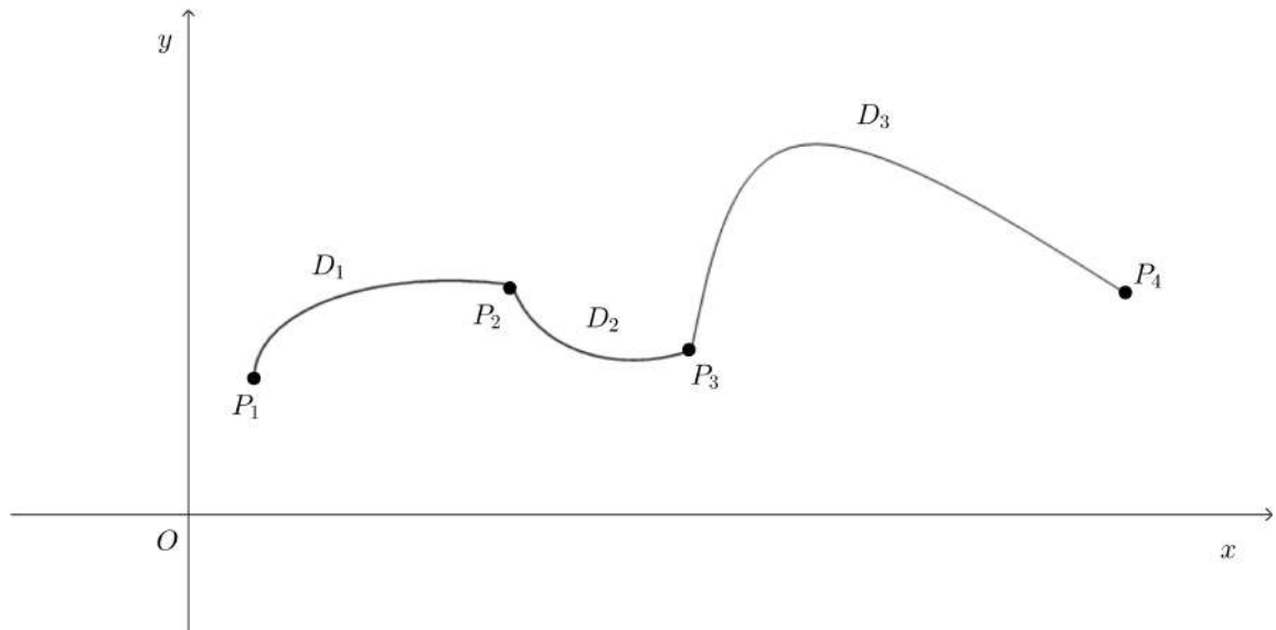
Figura 11 – Caminho D.
