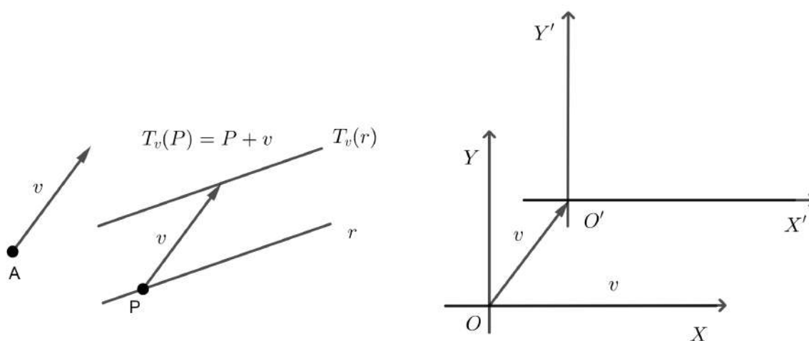
Figura 29 – Translação.
