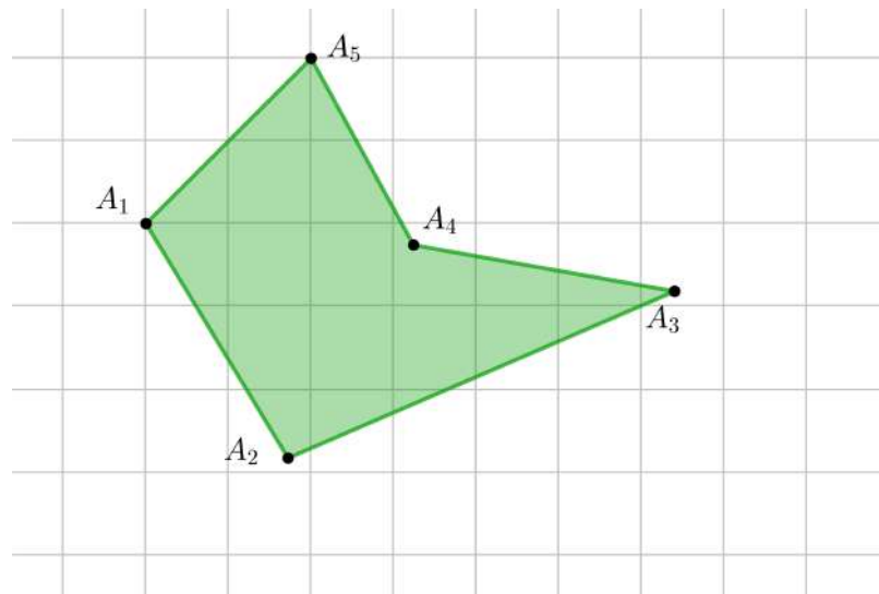
Figura 21 – Polígono A_1A_2A_3A_4A_5 .
