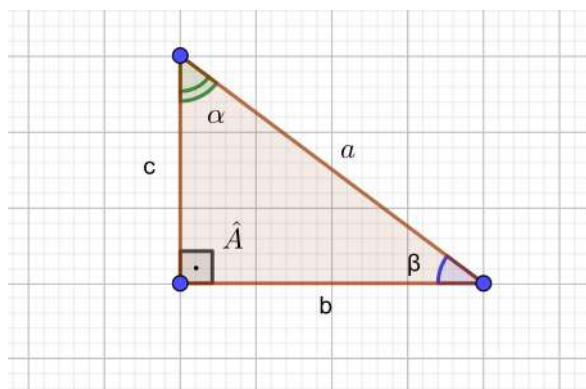
Figura 60 – Triângulo Retângulo.
