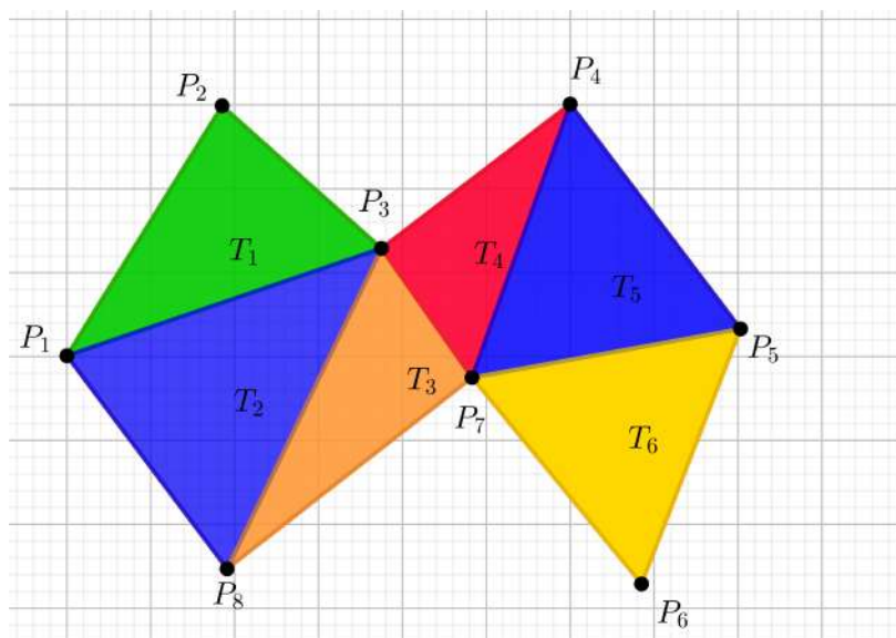
Figura 50 – Polígono: P_1P_2P_3P_4P_5P_6P_7P_8 .
