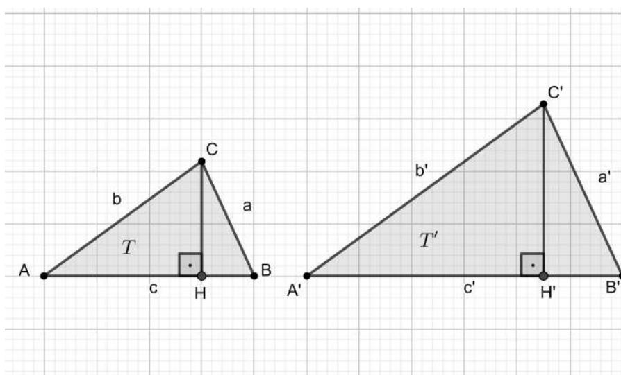
Figura 49 – Triângulos semelhantes.
