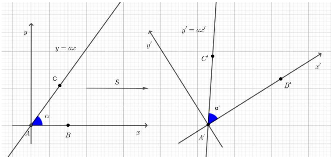
Figura 41 – Ângulos Congruentes
