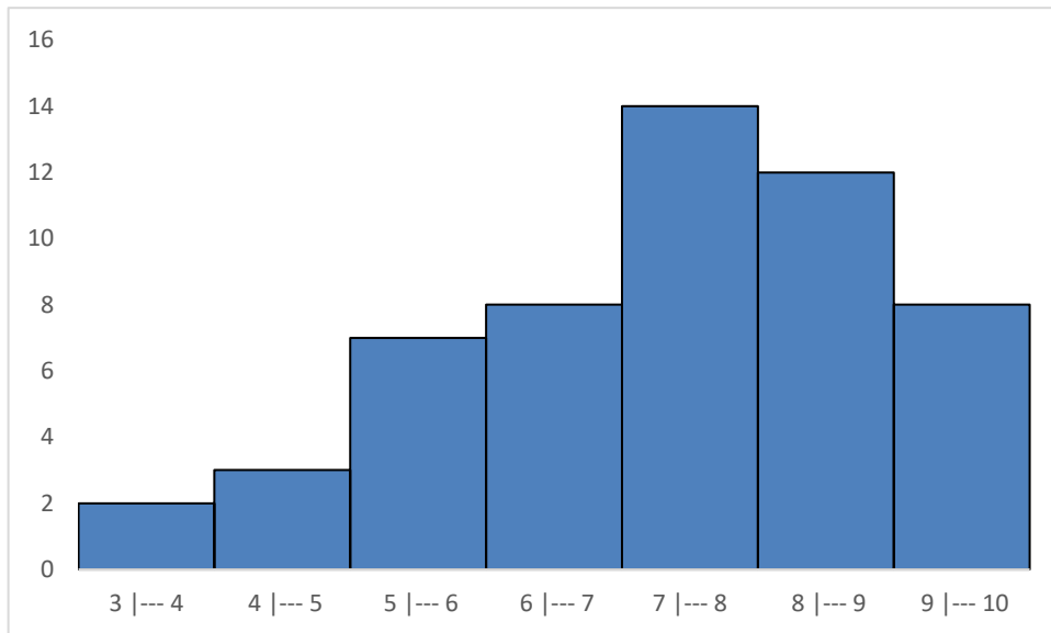
Figura 6-Exemplo de Histograma
